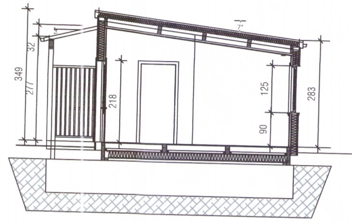
PVERSNIÐ A-A
