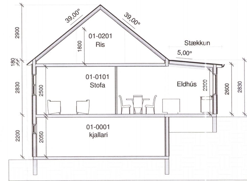
Snið A-A 1 : 100
