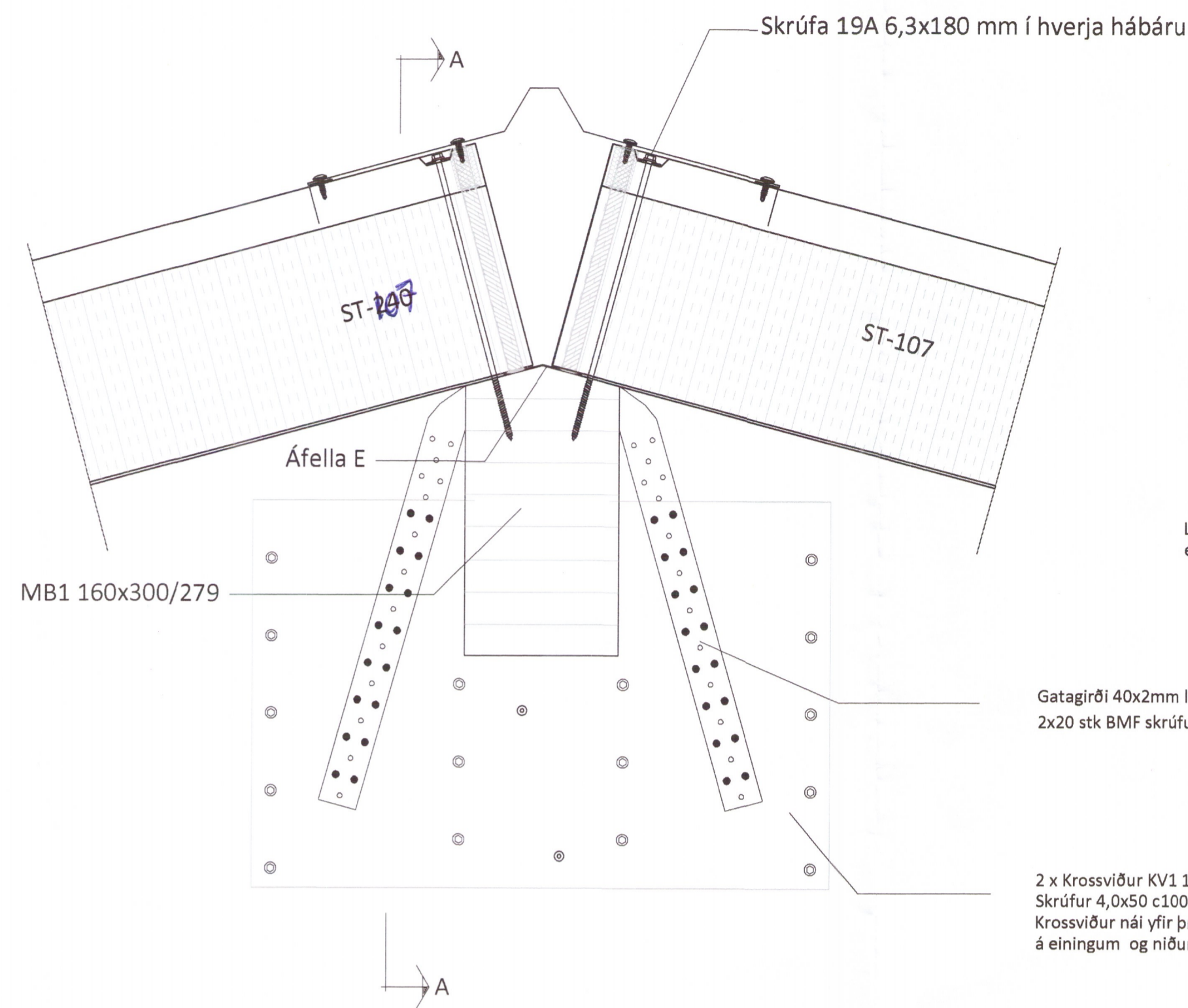
Sérmynd 1 Mkv. 1:5
