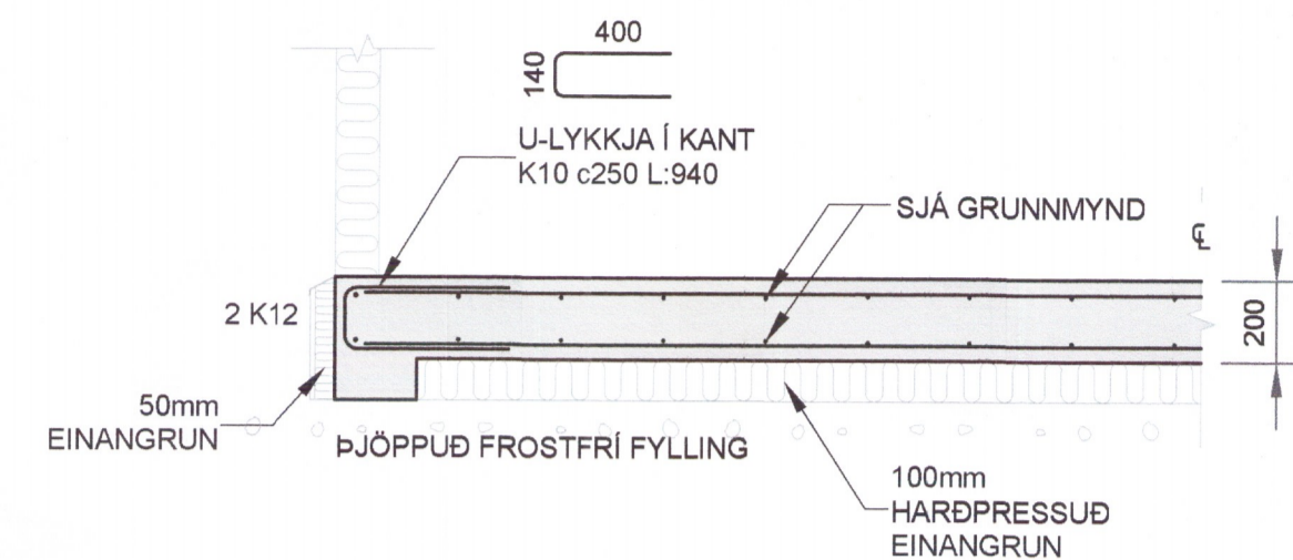
SNIÐ C Mkv. 1:20
