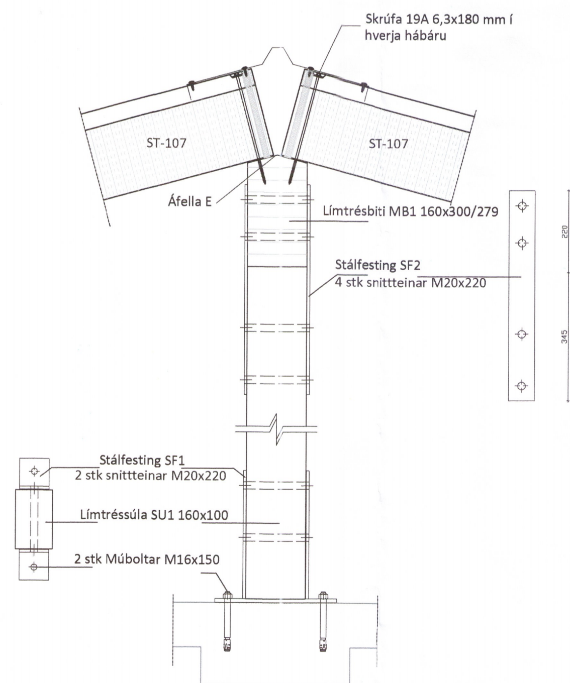
Sérmynd 4 Mkv. 1:10
