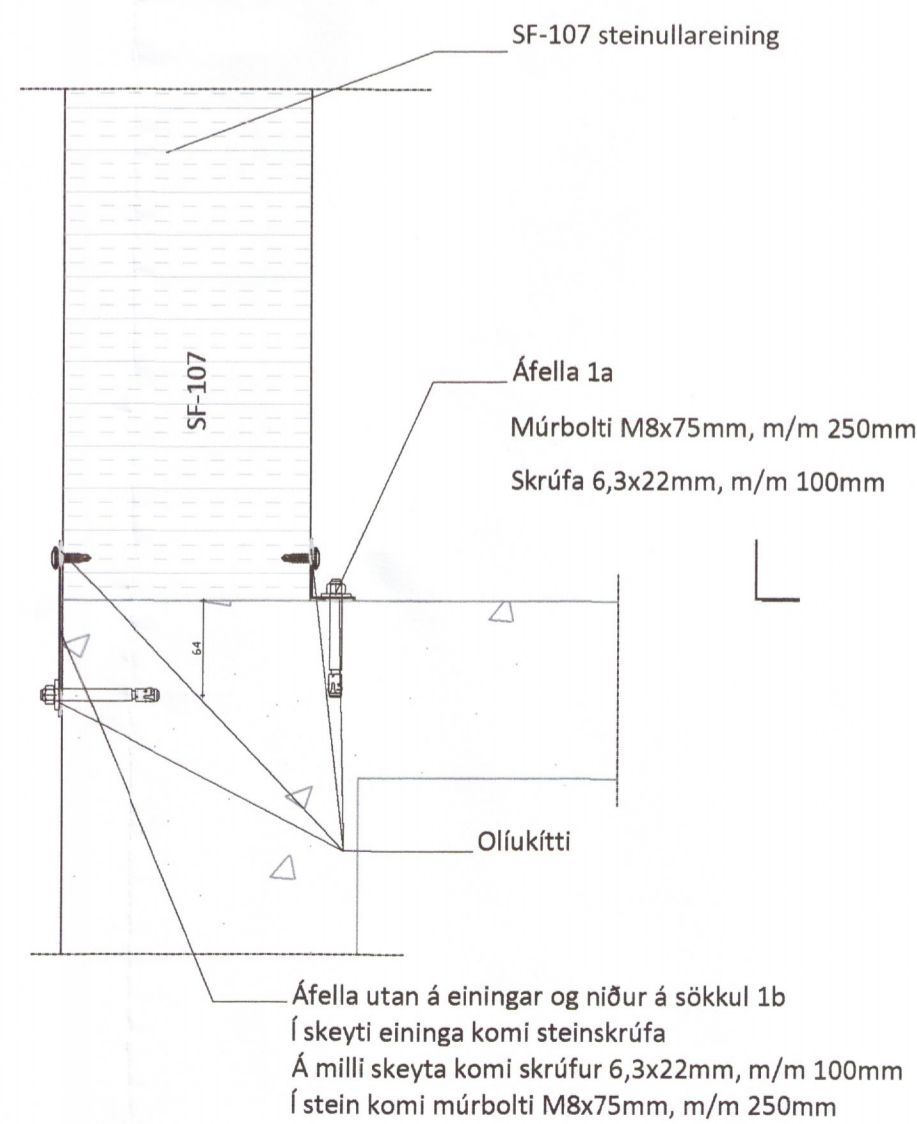
Sérmynd 3 Mkv. 1:5
