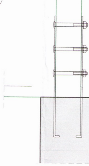
Deili 1:10
