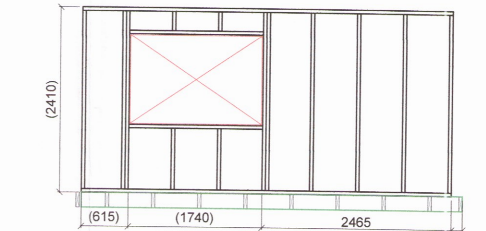
Veggjagrind 01 Mkv. 1:50
