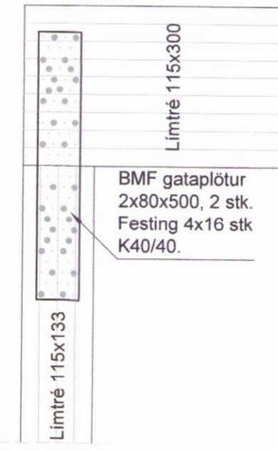
Snið 1:10
