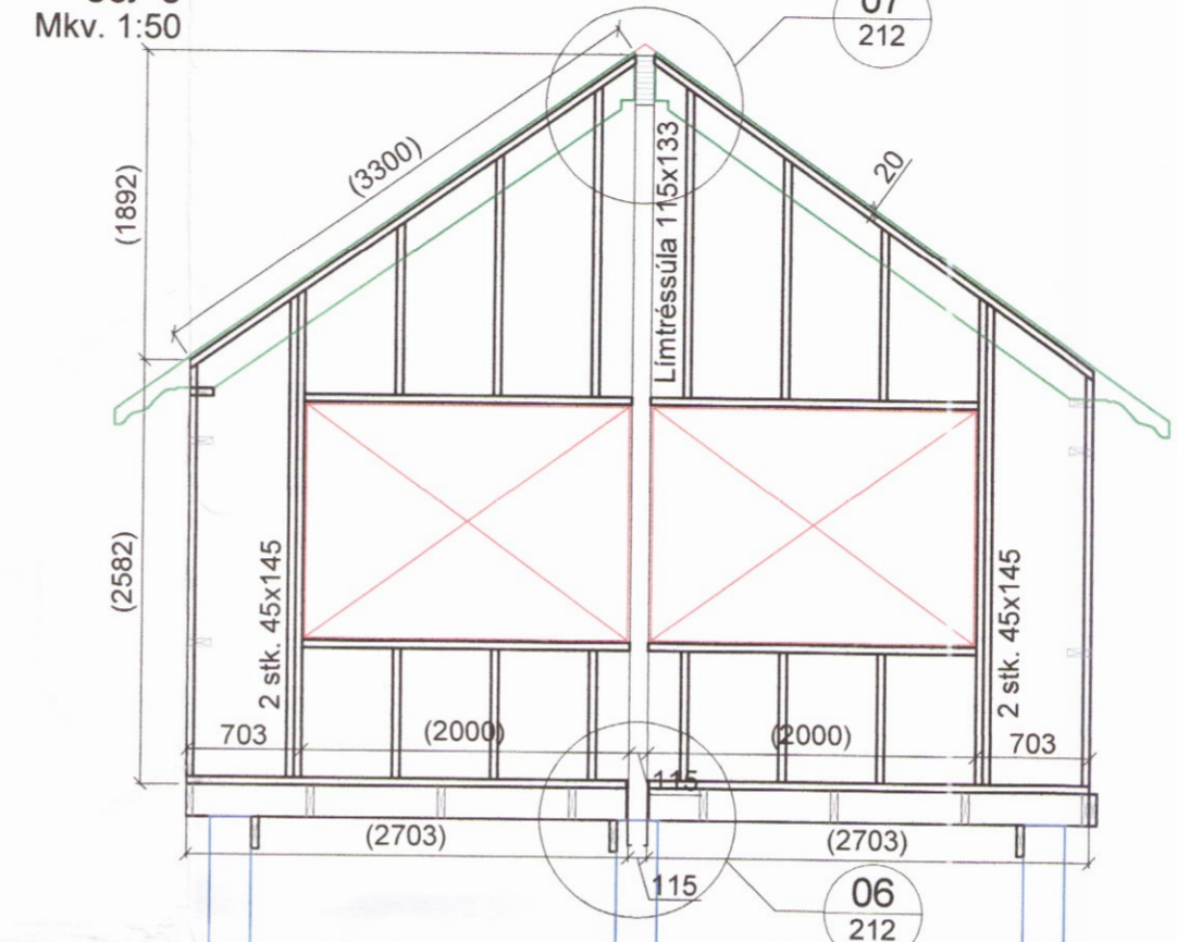
Veggjagrind 02 Mkv. 1:50
