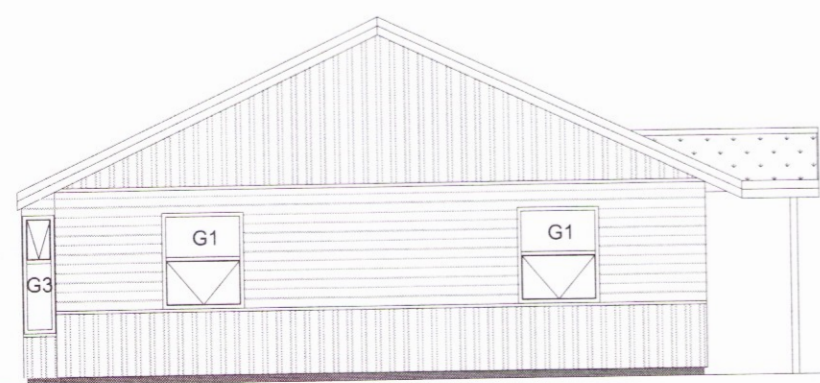
ÚTLIT - NORÐUR
