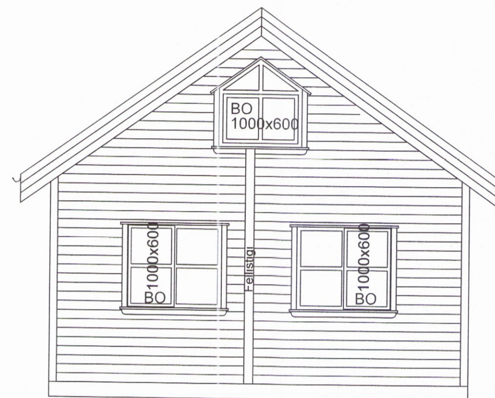
Suður 1:50
