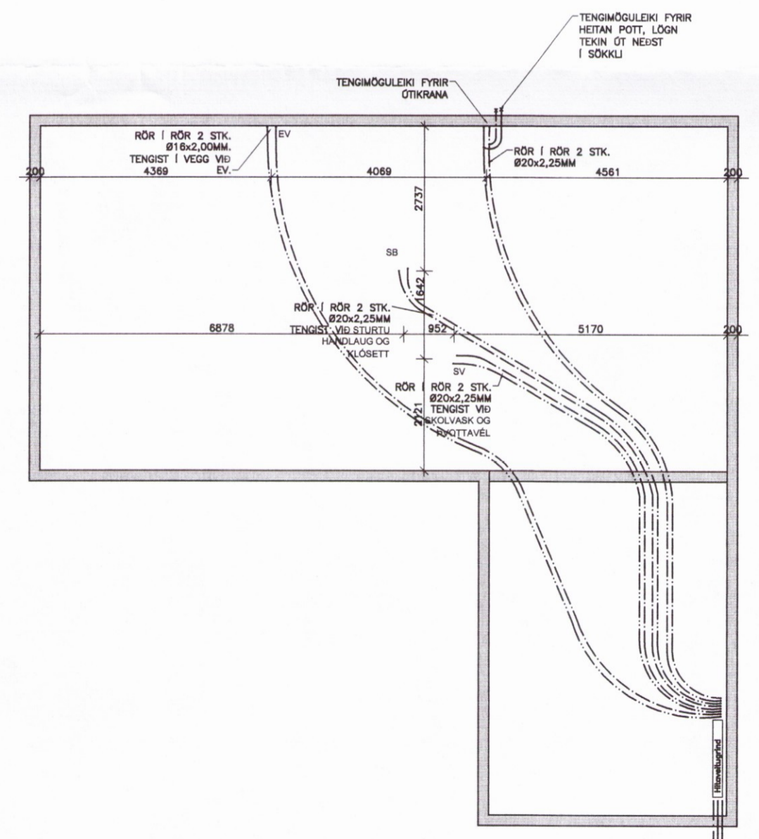
GRUNNMYND GRUNNVATNSLAGNIR 1:50 LYNGBREKKA NR. 5
