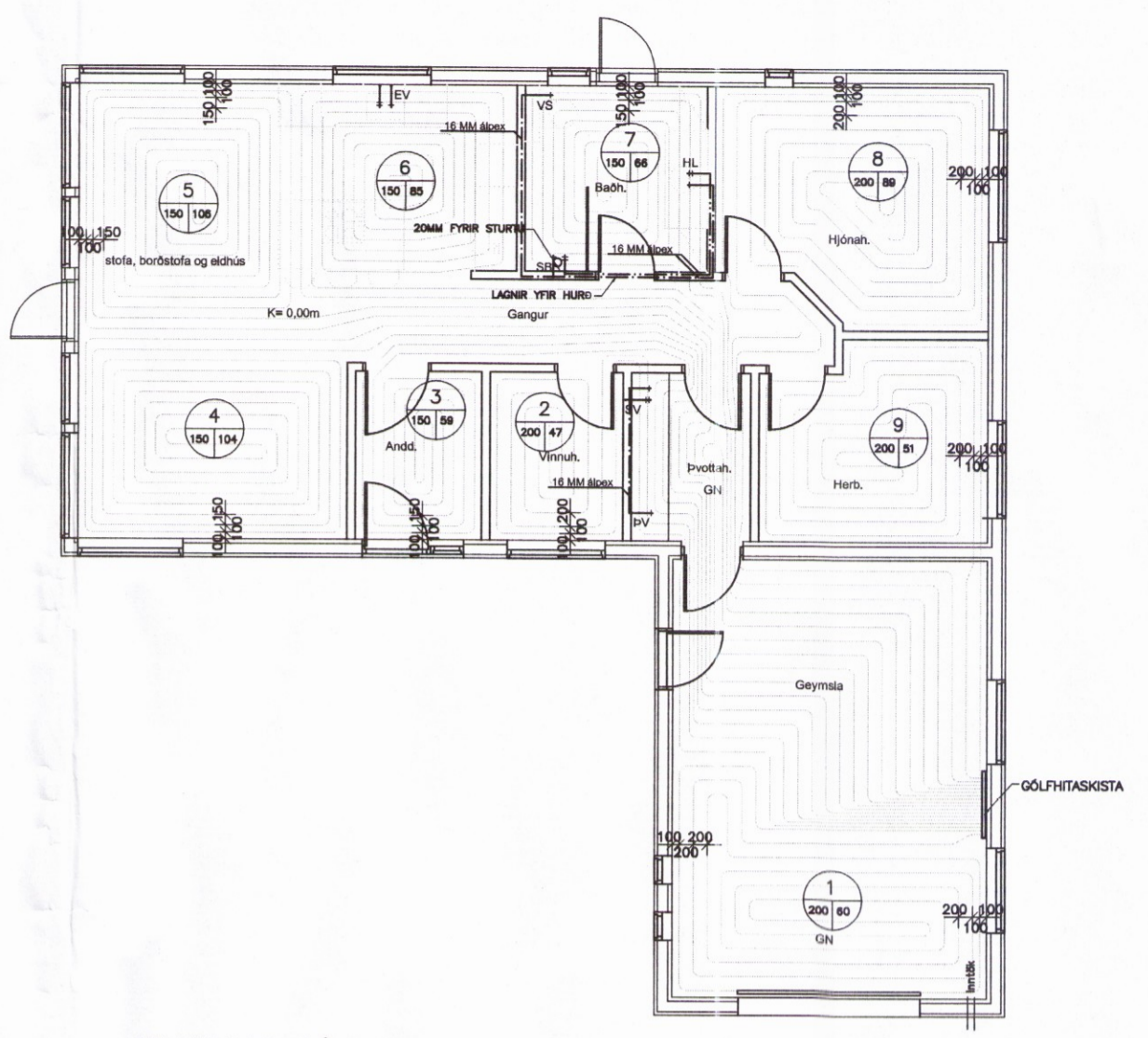
GRUNNMYND GÖLFHITA- OG NEYSLUVATNSLAGNIR 1:50 LYNGBREKKA NR. 5
