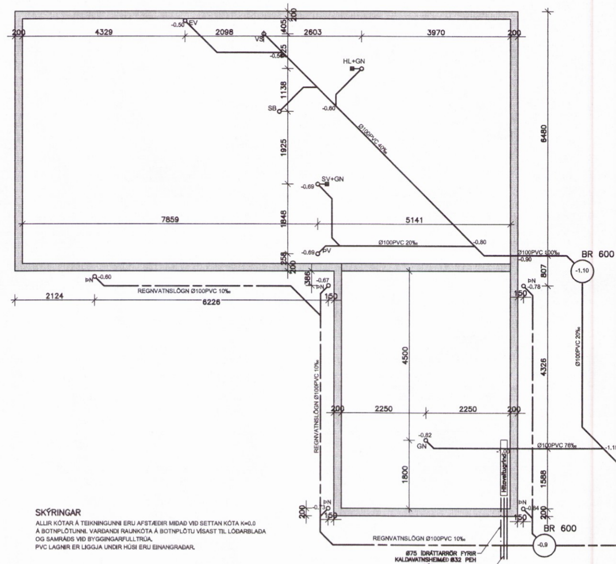
GRUNNMYND GRUNNVATNSLAGNIR 1:50 LYNGBREKKA NR. 5
