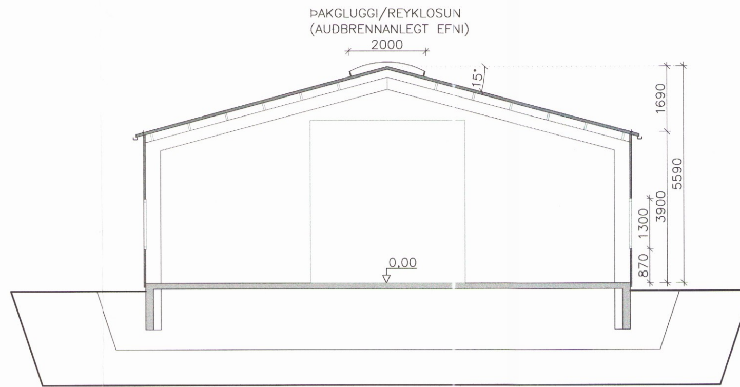
SNEIDING A 1:100
