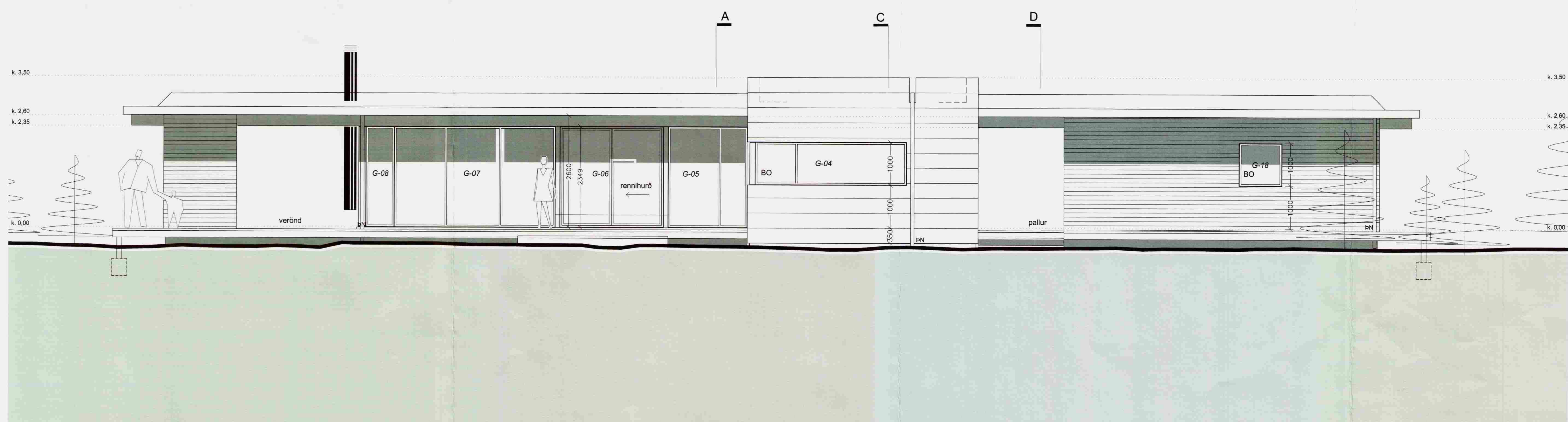
ÚTLIT SUÐAUSTUR M 1:50
