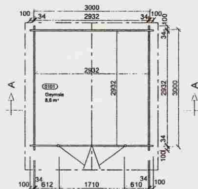
GRUNNMYND
