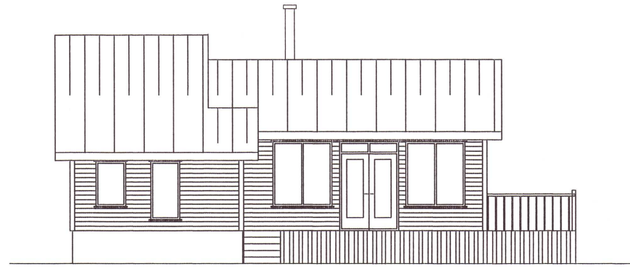
Suðurhlíð M. 1:100
