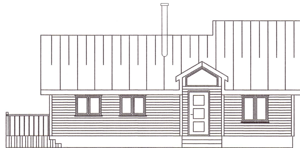
Norðurhlíð M. 1:100
