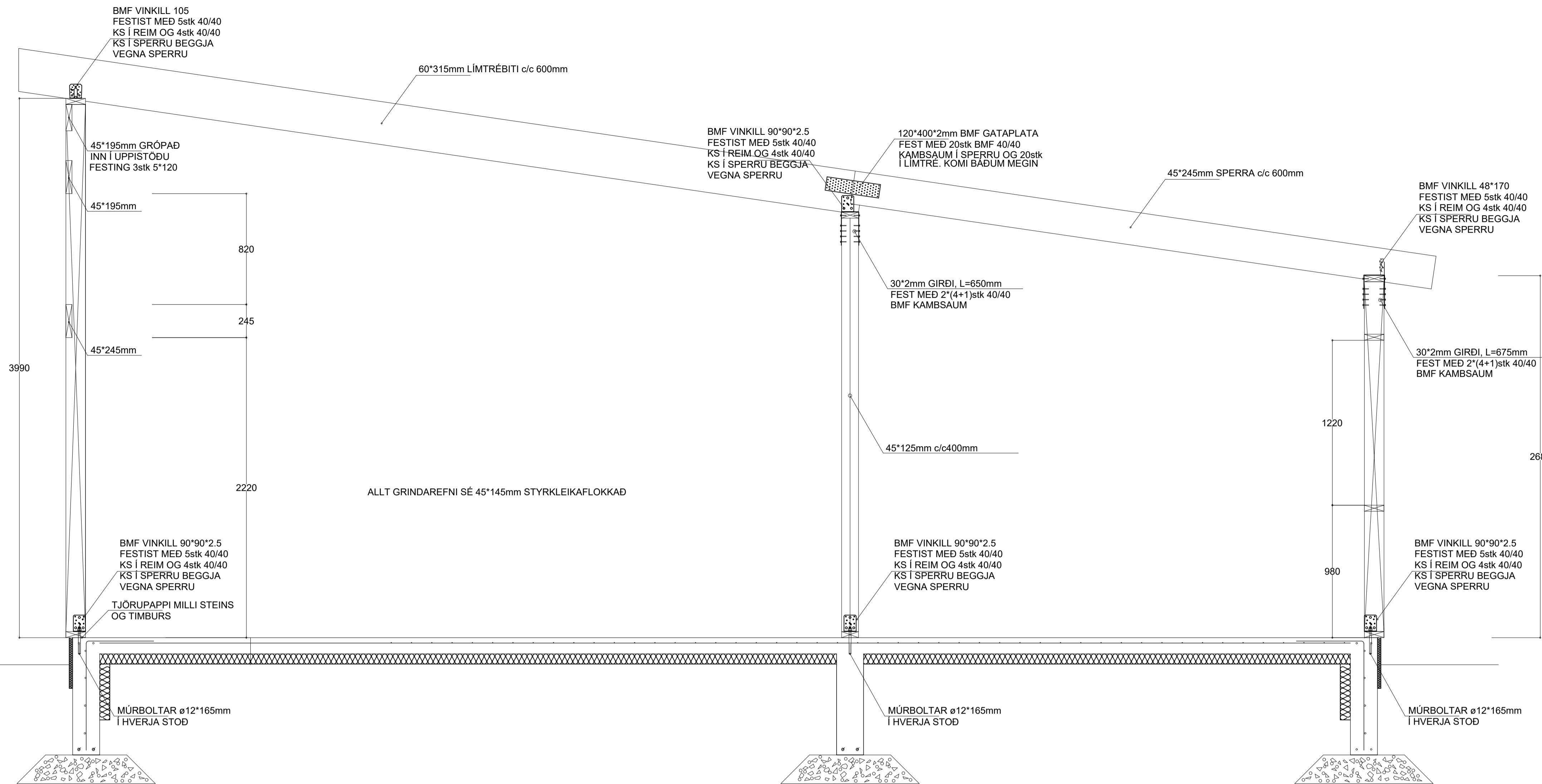
SNEIÐING B - mkv. 1:20
