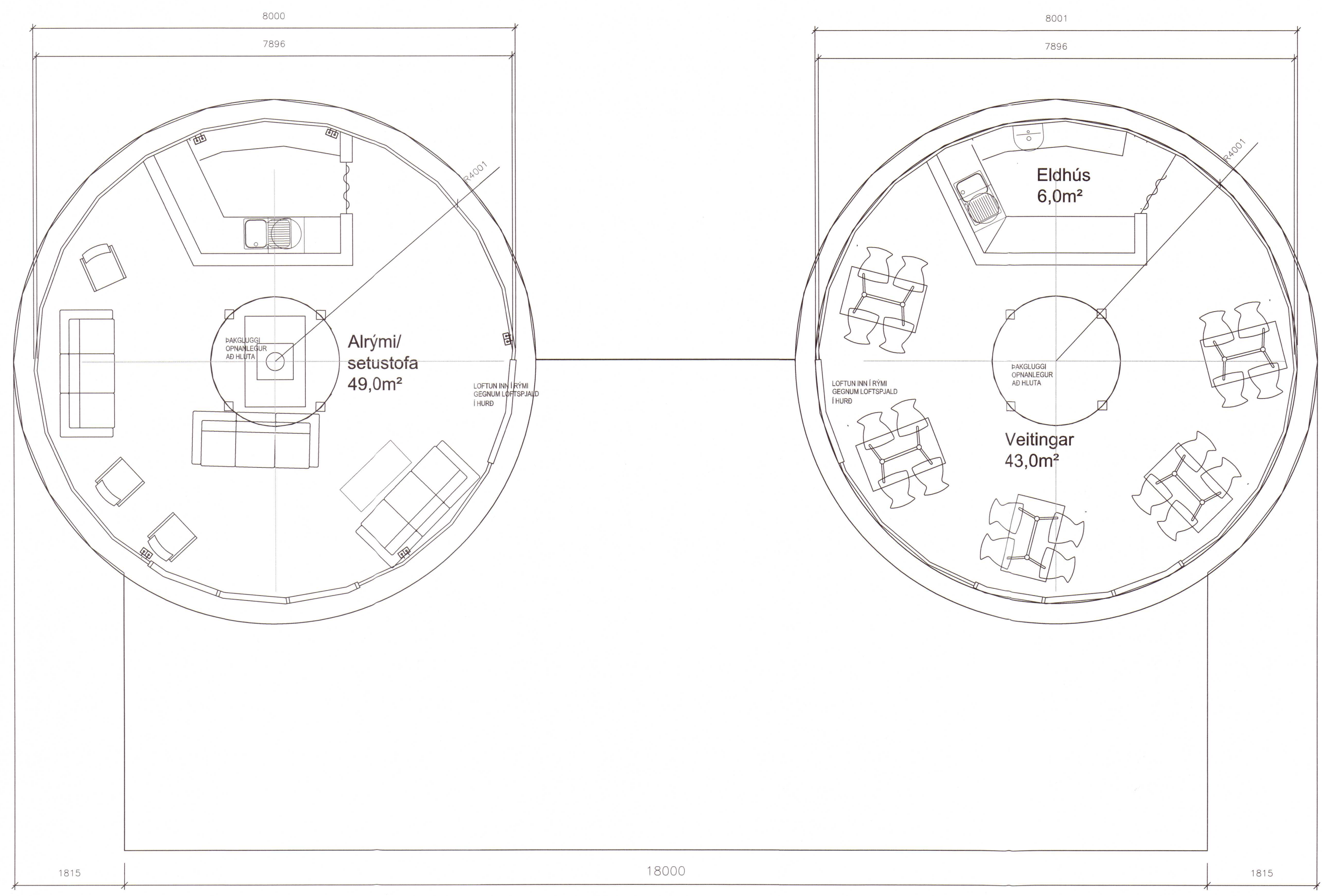
GRUNNMYND ÞJÓNUSTUTJALD 1:50
