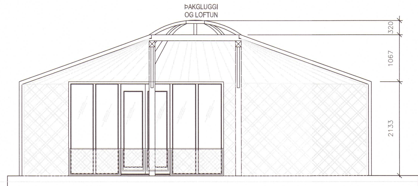
SNÍÐ 1:50
