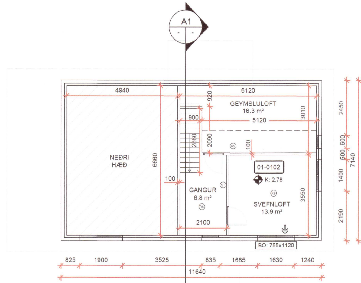
GRUNNMYND SVEFNLOFT Mkv. 1:100
