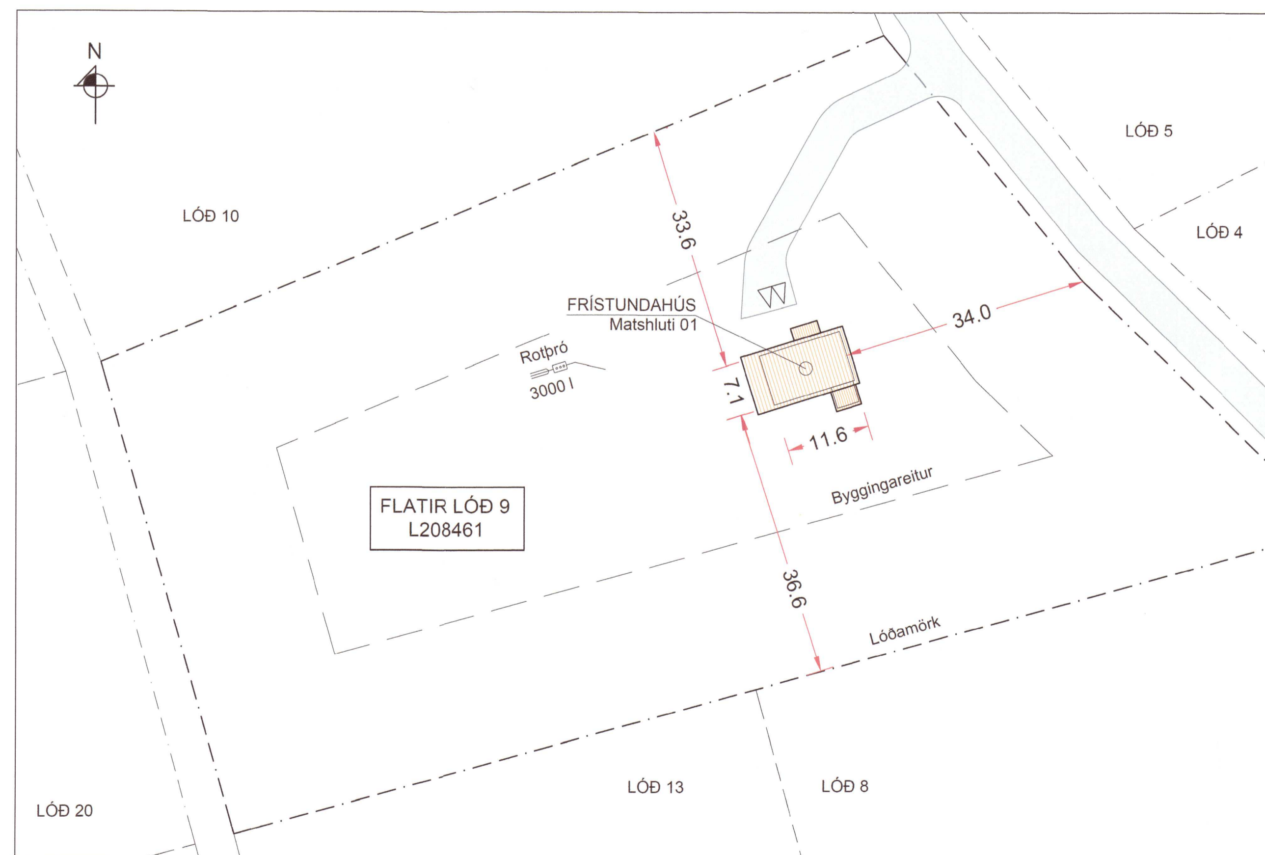
AFSTÖDUMYND Mkv. 1:500
