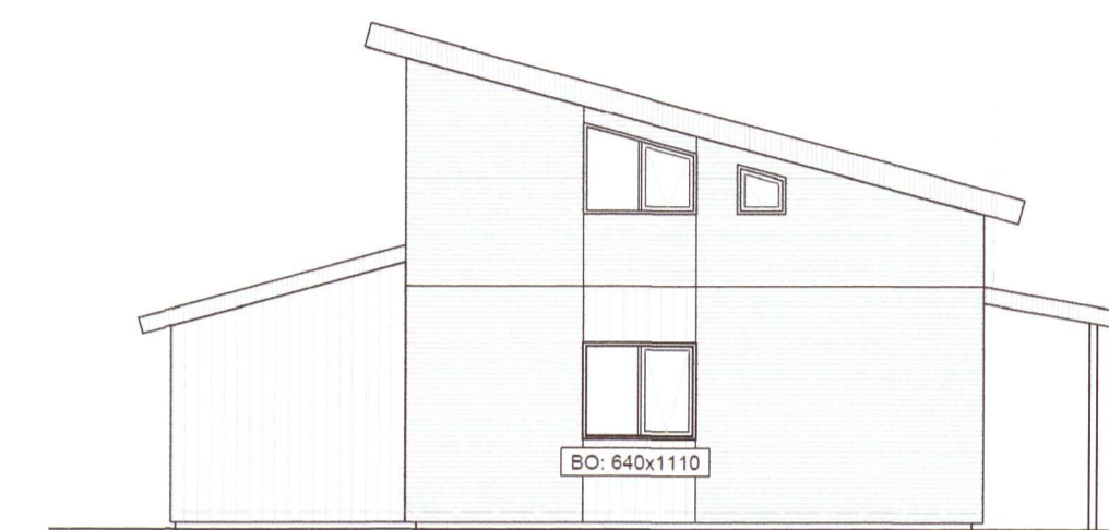
ÚTLIT AUSTUR Mkv. 1:100
