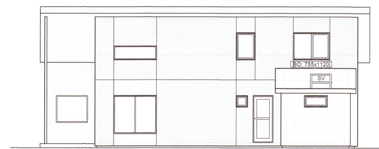
ÚTLIT SUÐUR Mkv. 1:100
