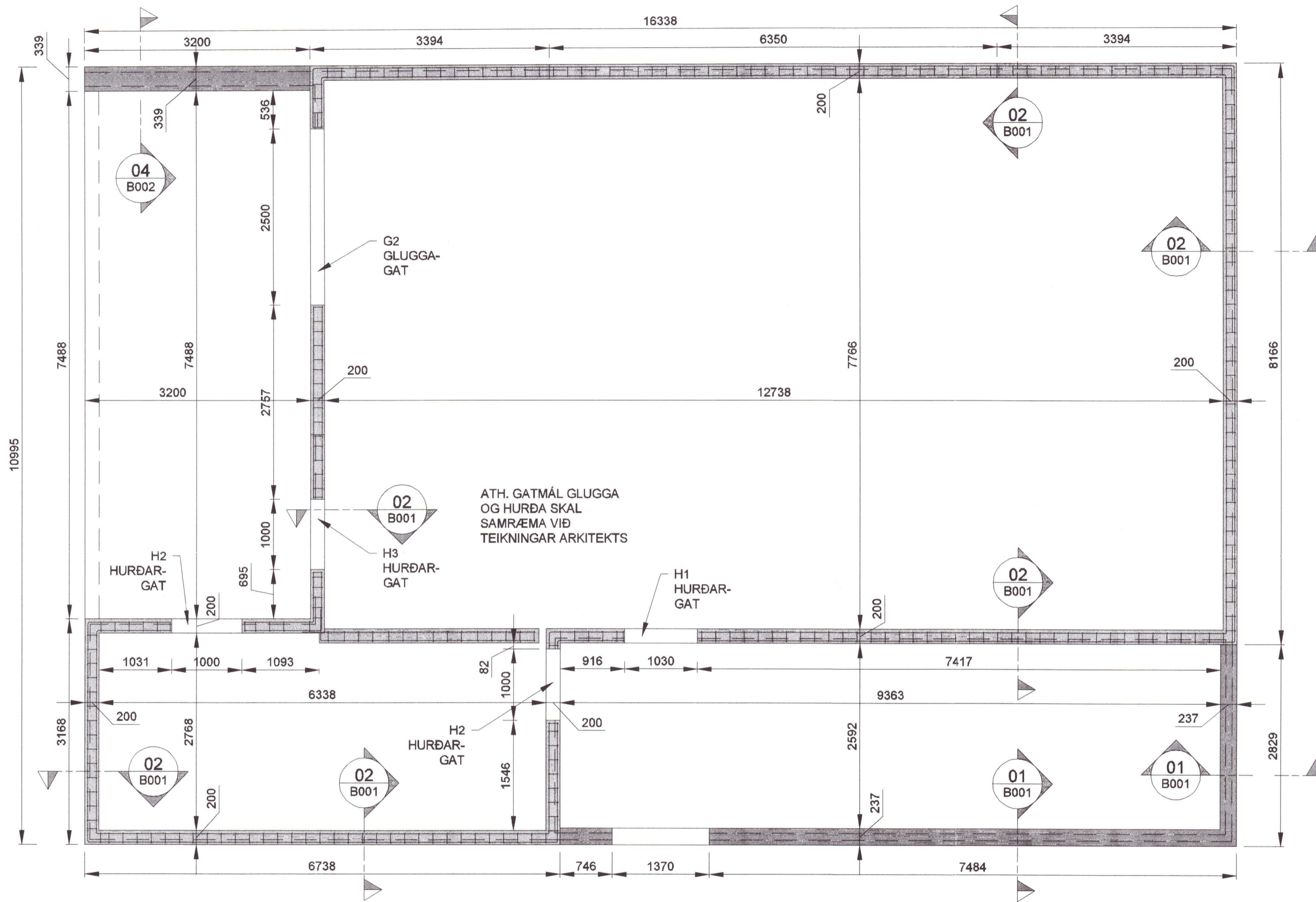
GRUNNMYND - ST.STEYPTIR VEGGIR 1:50 (A1)
