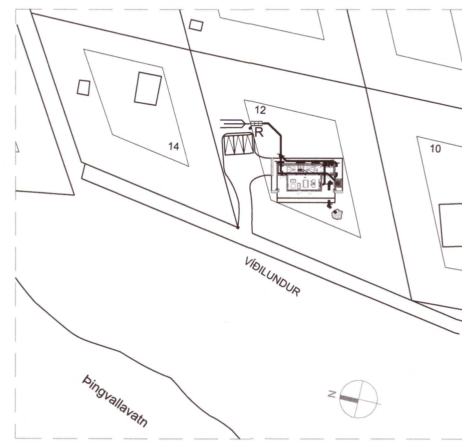
Afstöðumynd Mkv. 1:1000
