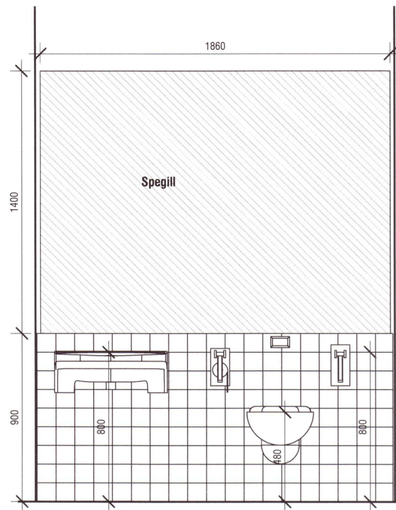
1 Salerni 1 : 20
