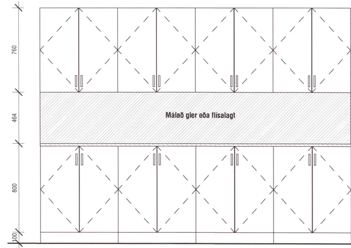
2 Eldhúsinnrétting 1 : 20
