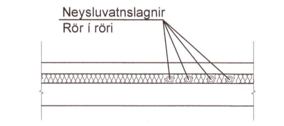
A SNÍÐ 1:20
