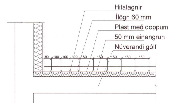
B SNÍÐ 1:20
