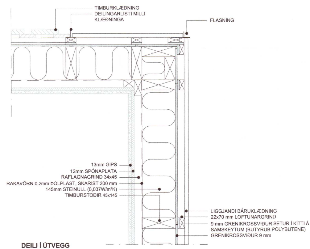
DEILI Í ÚTVEGG 1:10
