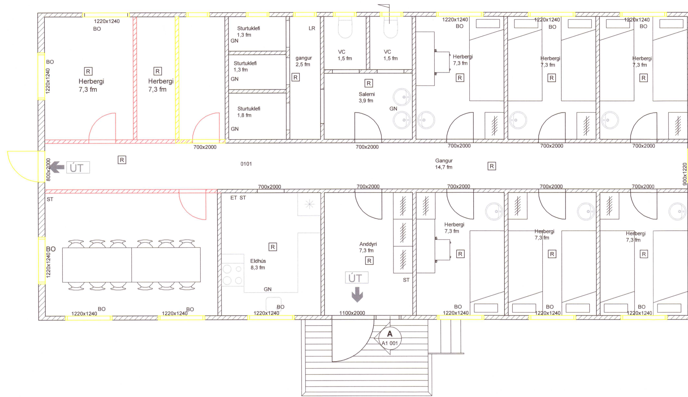
Grunnmynd 1.hæð 1:50
