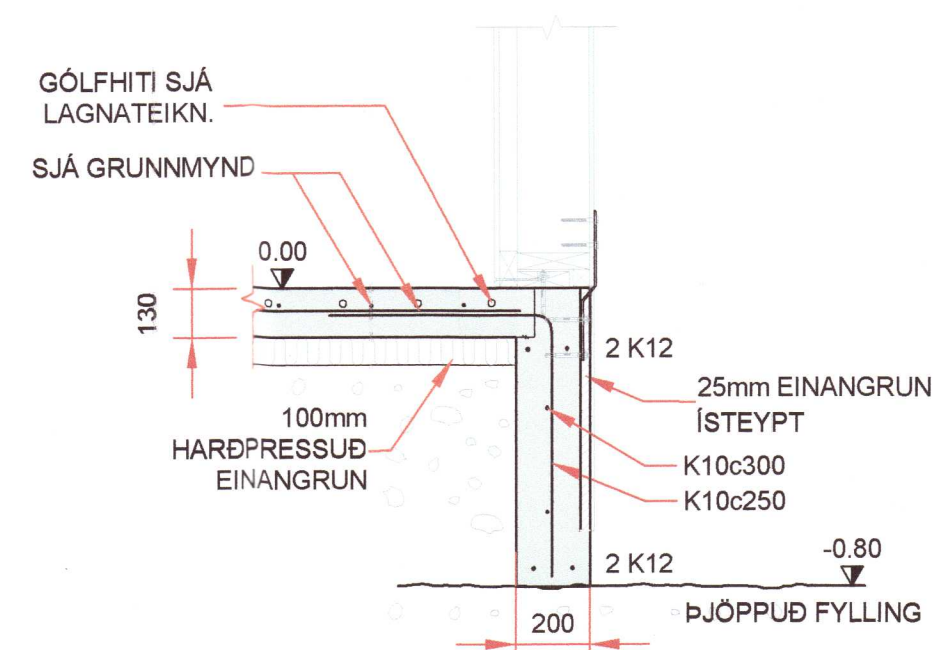
SNID 01 Mkv. 1:20
