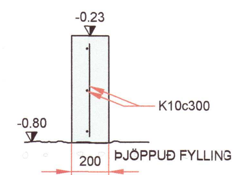
SNID 02 Mkv. 1:20
