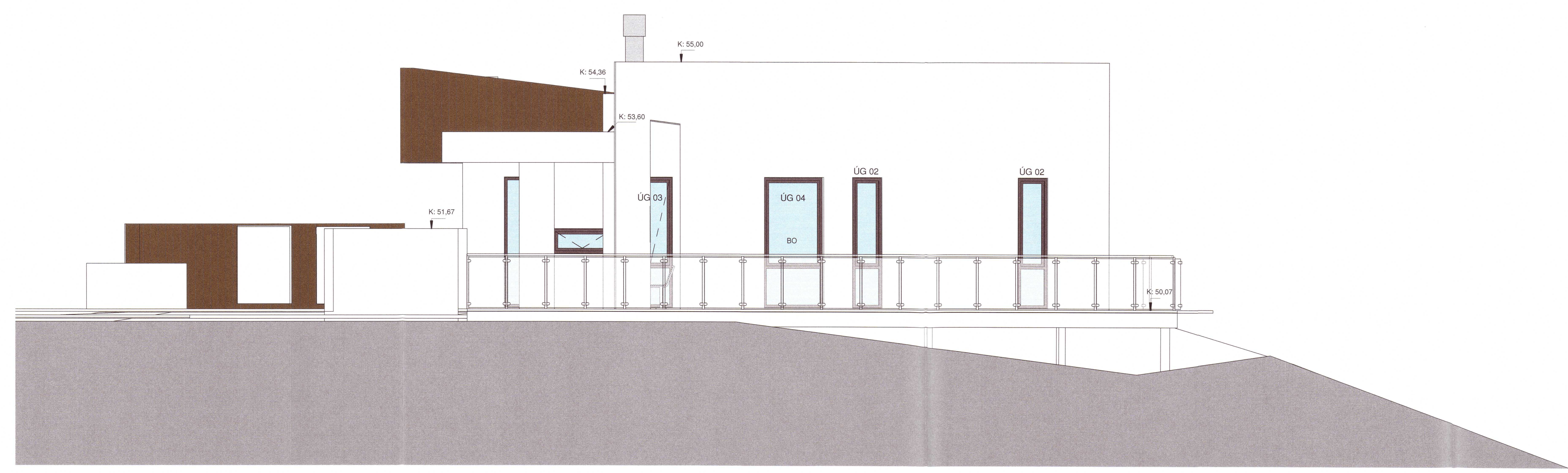
2 Útlit suður 1/50 1 : 50
