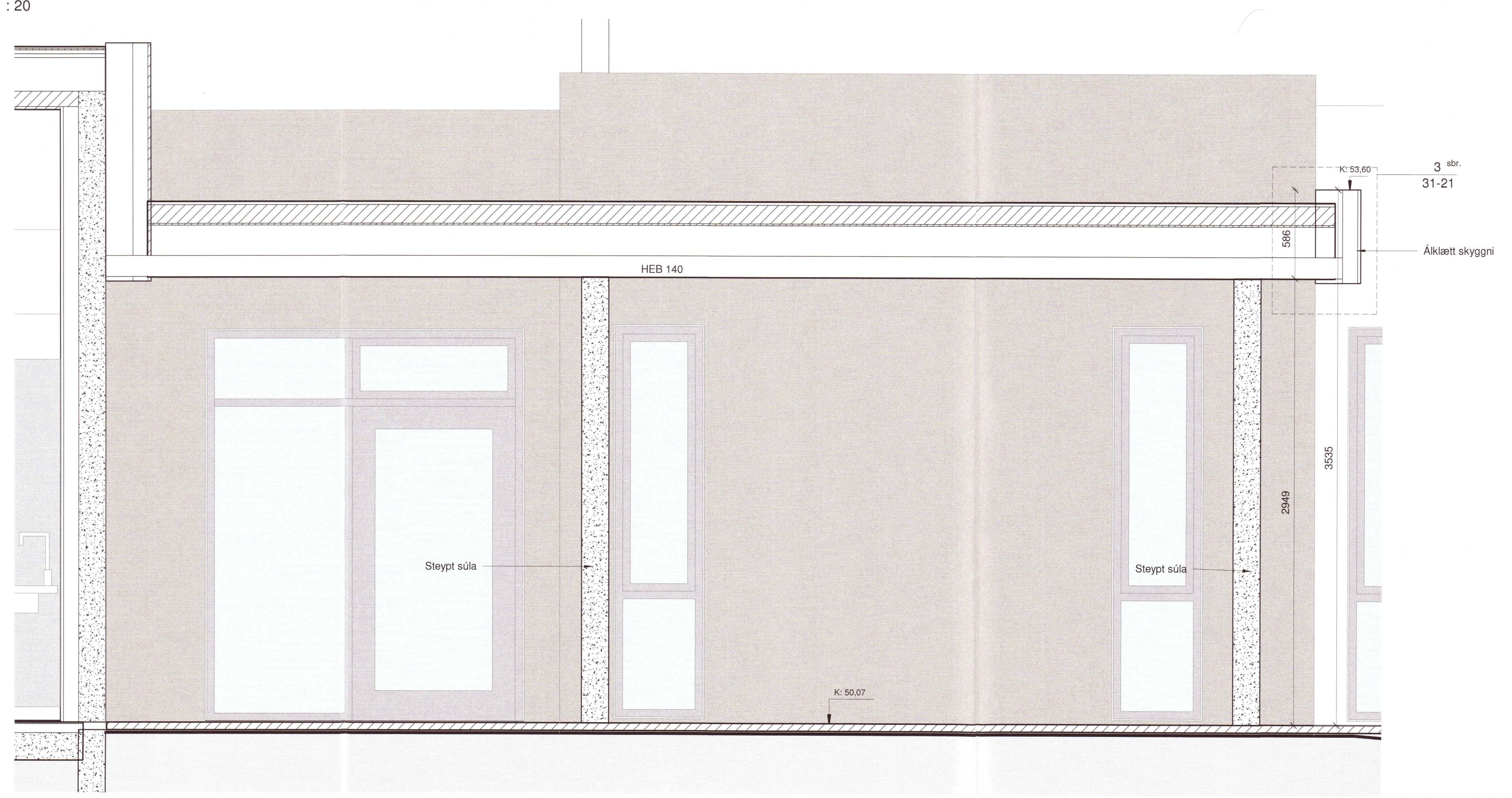
2 Skyggni yfir inngang - Snið B 1 : 20
