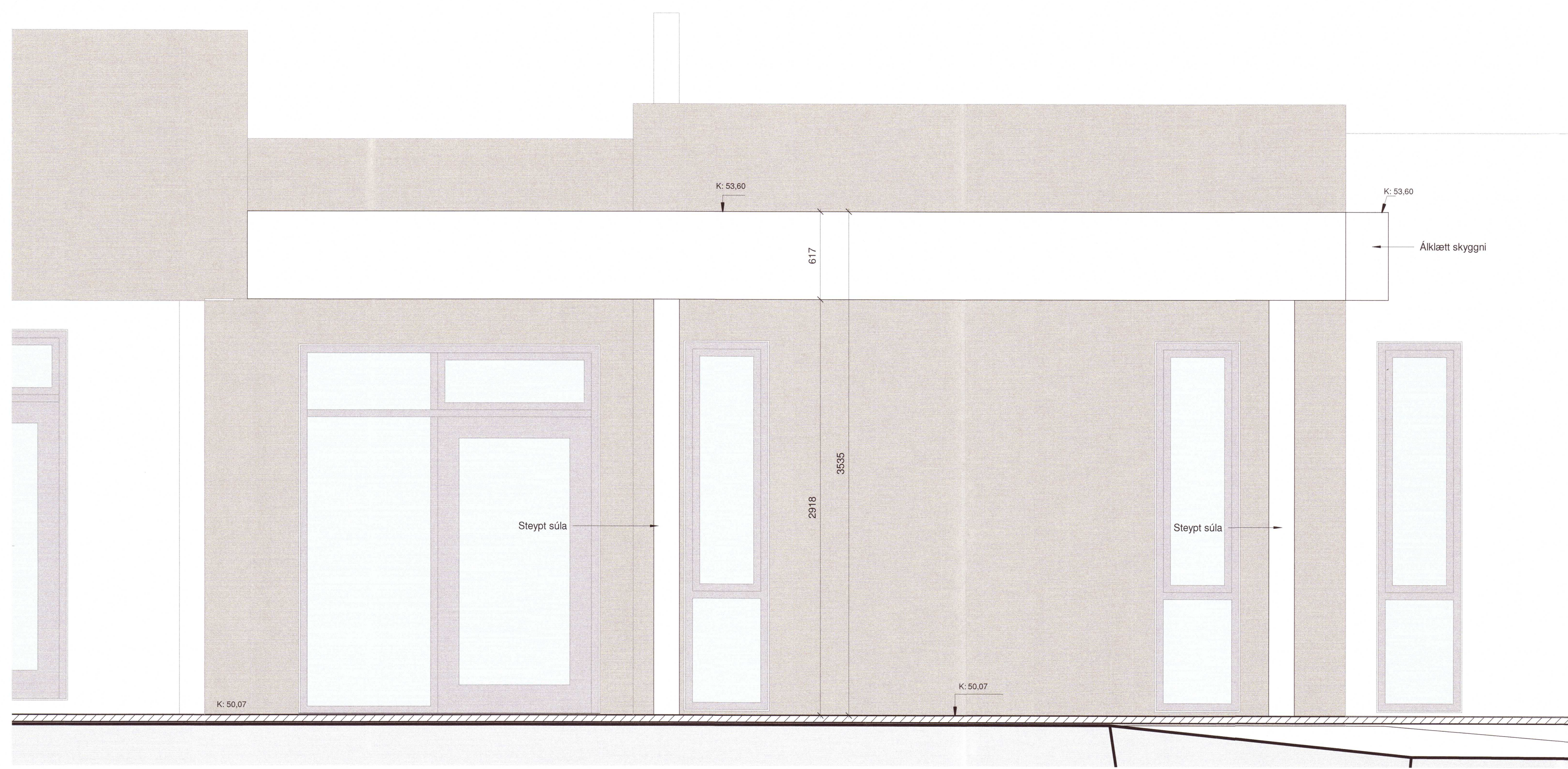
1 Skyggni útlit vestur 1 : 20
