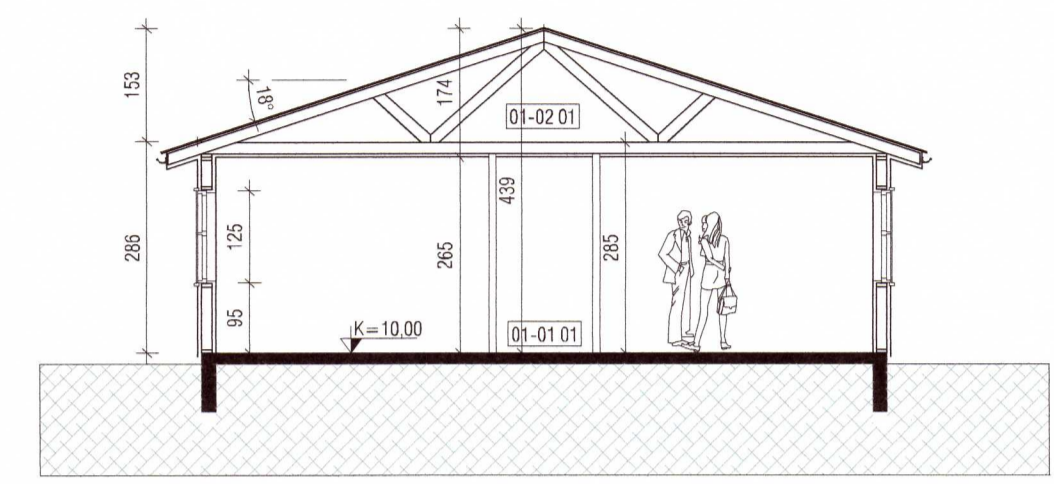
SNID A-A 1:100
