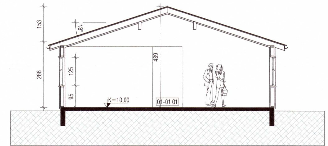
SNID B-B 1:100
