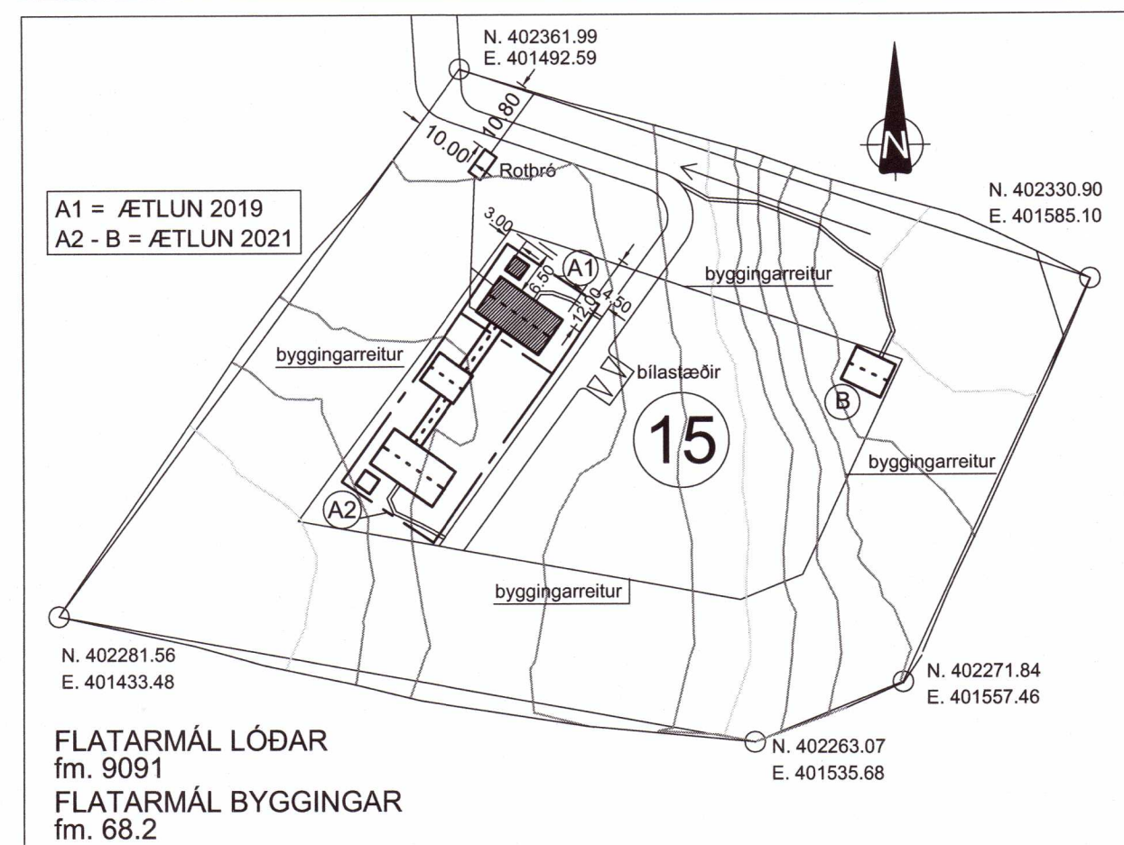
Afstöðumynd 1:1000
