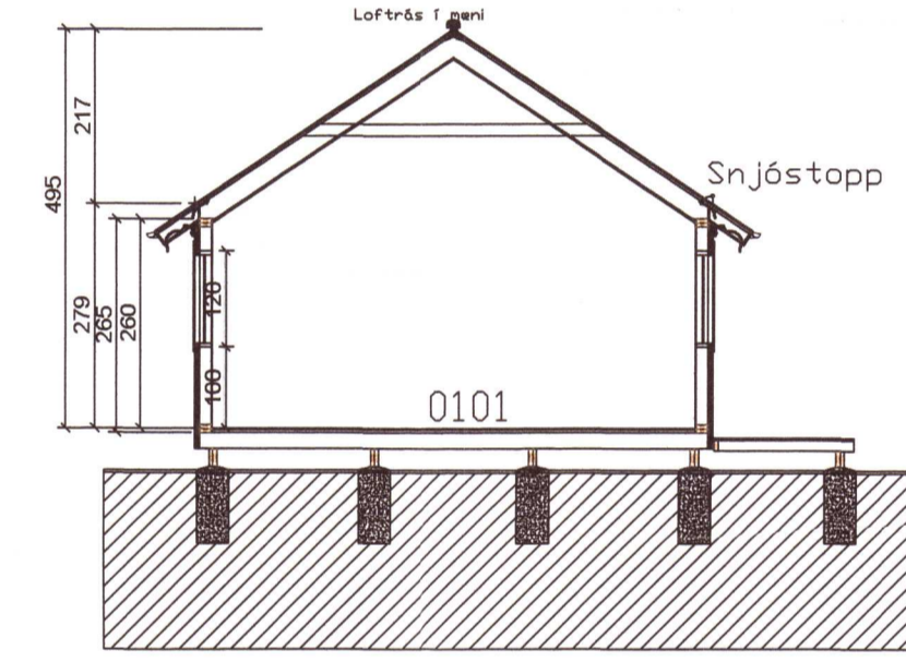
Snið B-B 1:100
