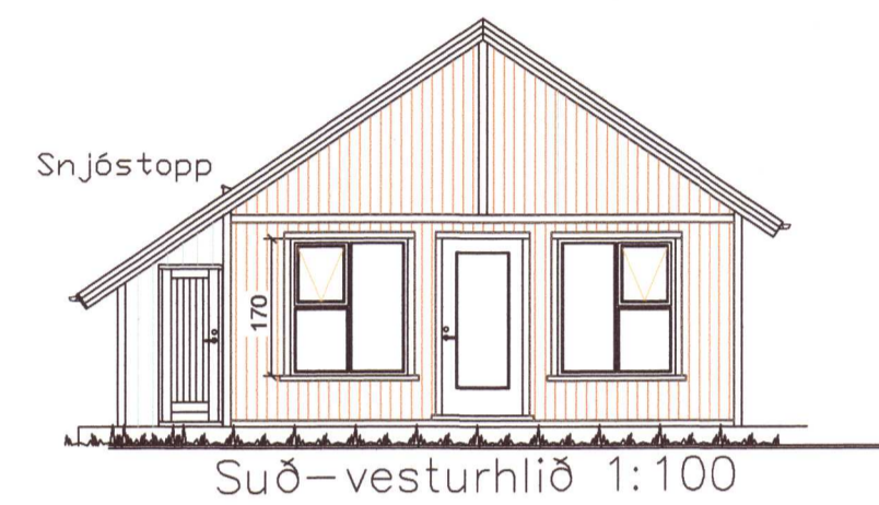
Suð-vesturhlíð 1:100
