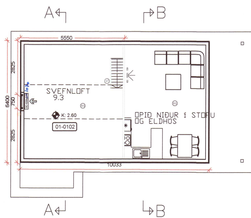
Svefnloft Grunnmynd 1:100
