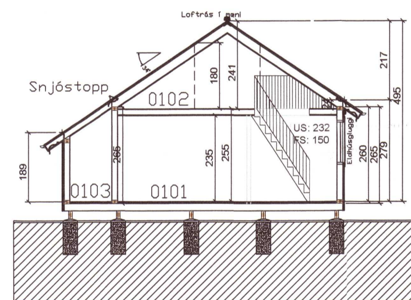
Snið A-A 1:100
