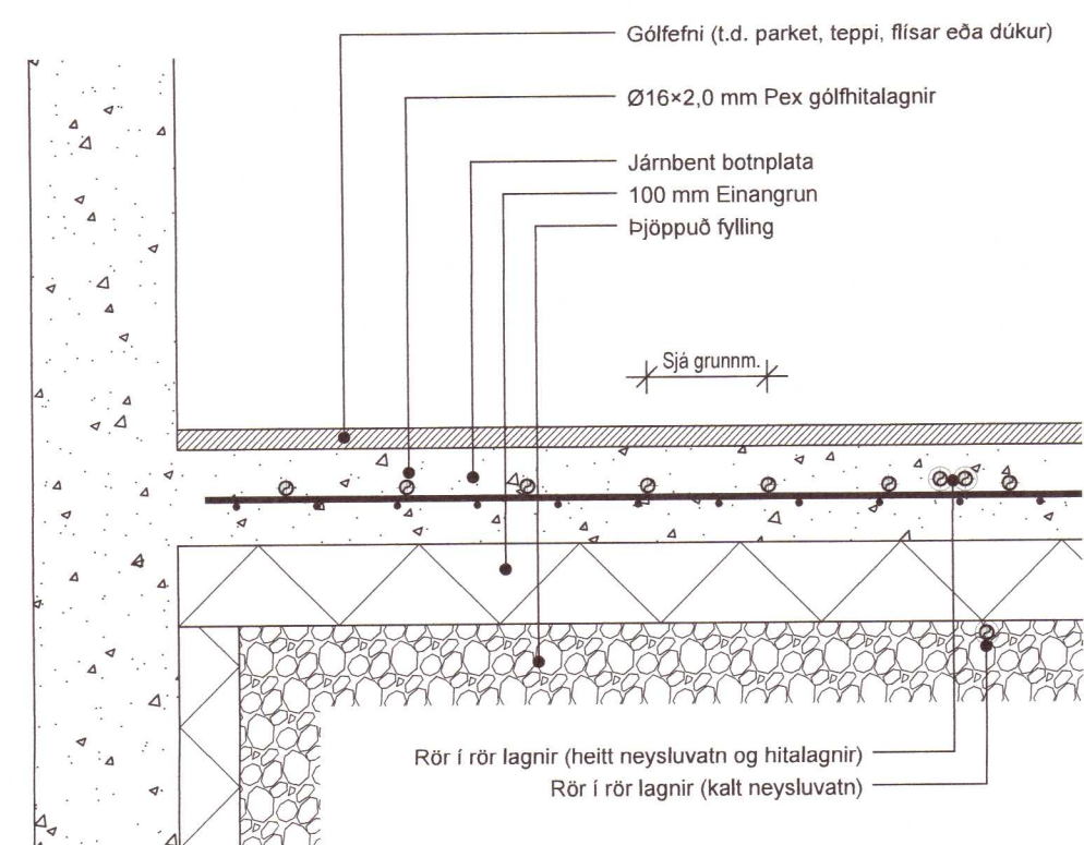
KENNISNIÐ GÓLFHITA 1:10
