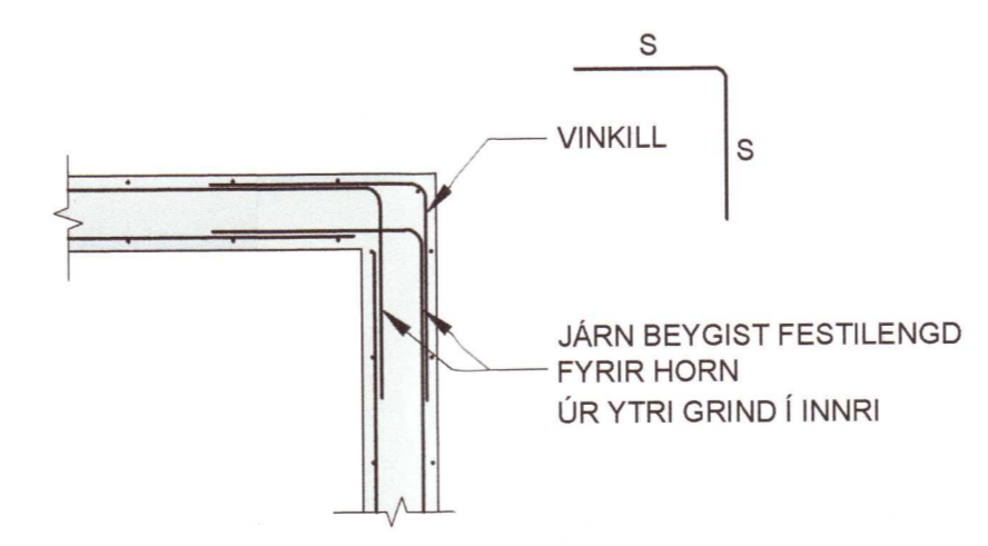
LÁRÉTT SNIÐ Í VEGGHORN Mkv 1:20
