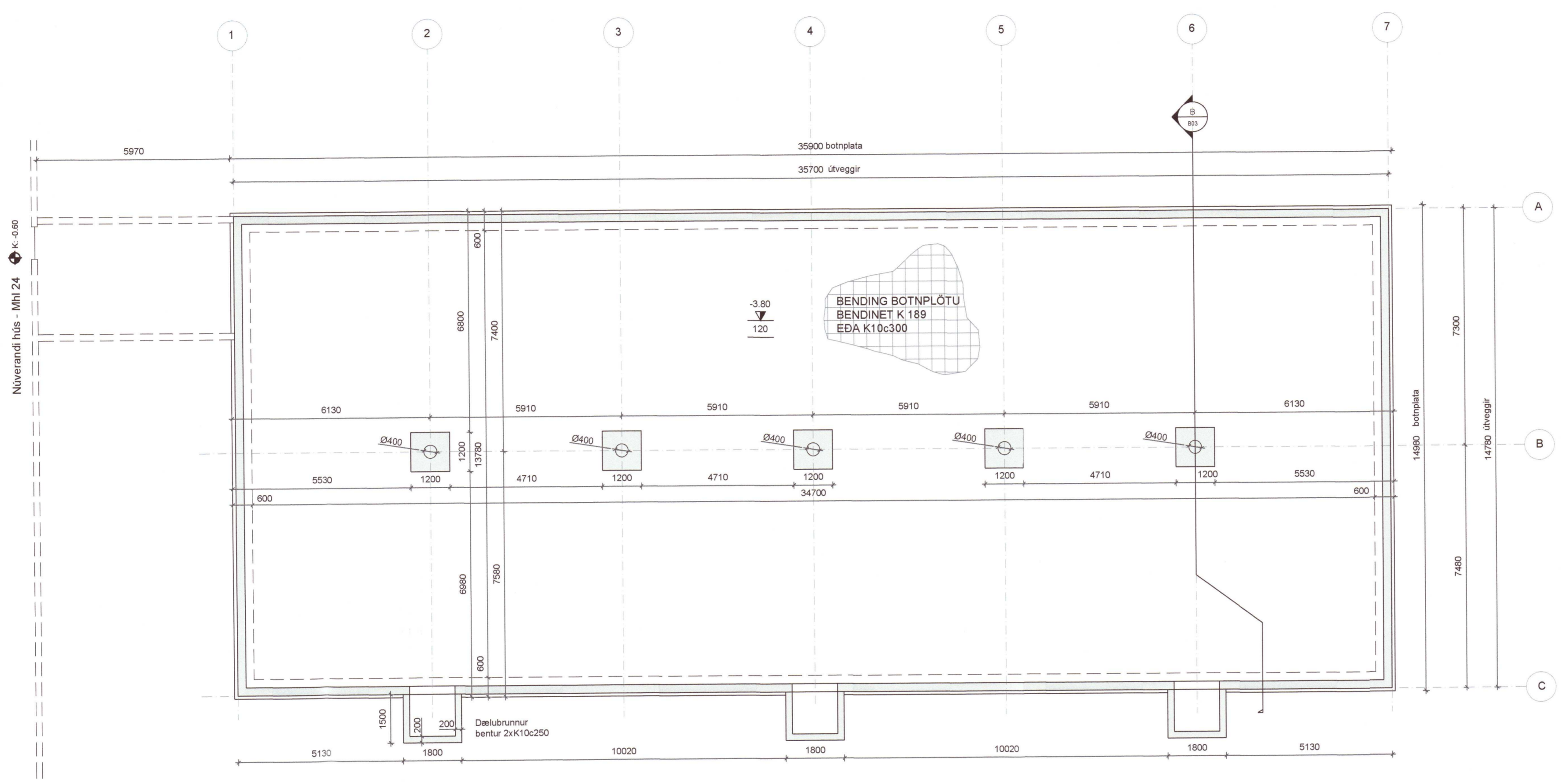
GRUNNMYND ÁBURÐARKJALLARA MKV. 1:100
