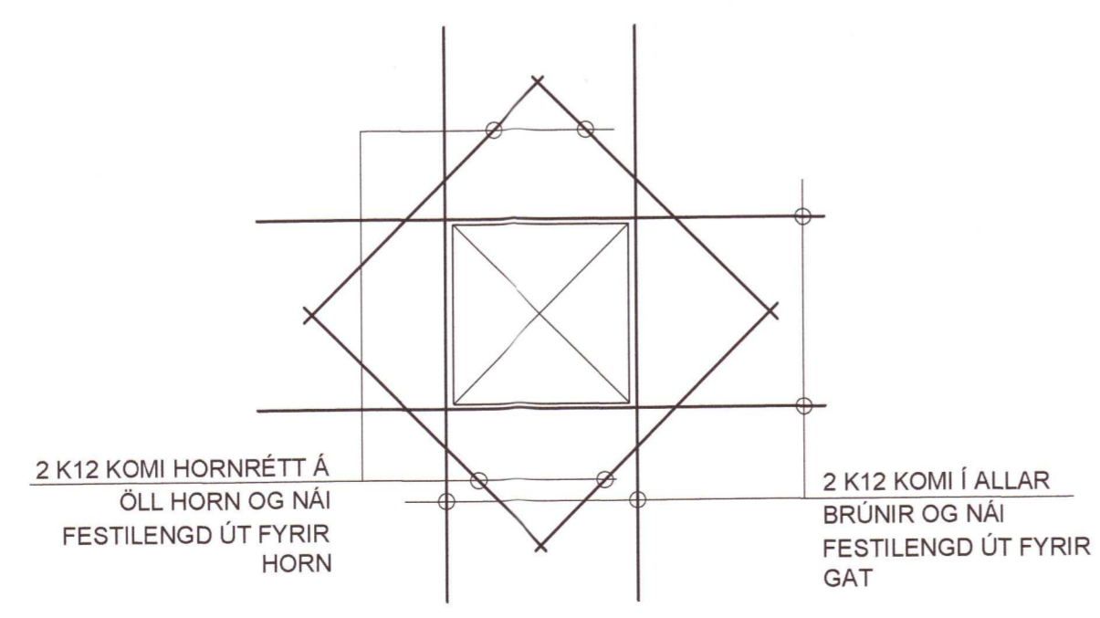
BENDING Í KRING UM OP Mkv 1:20
