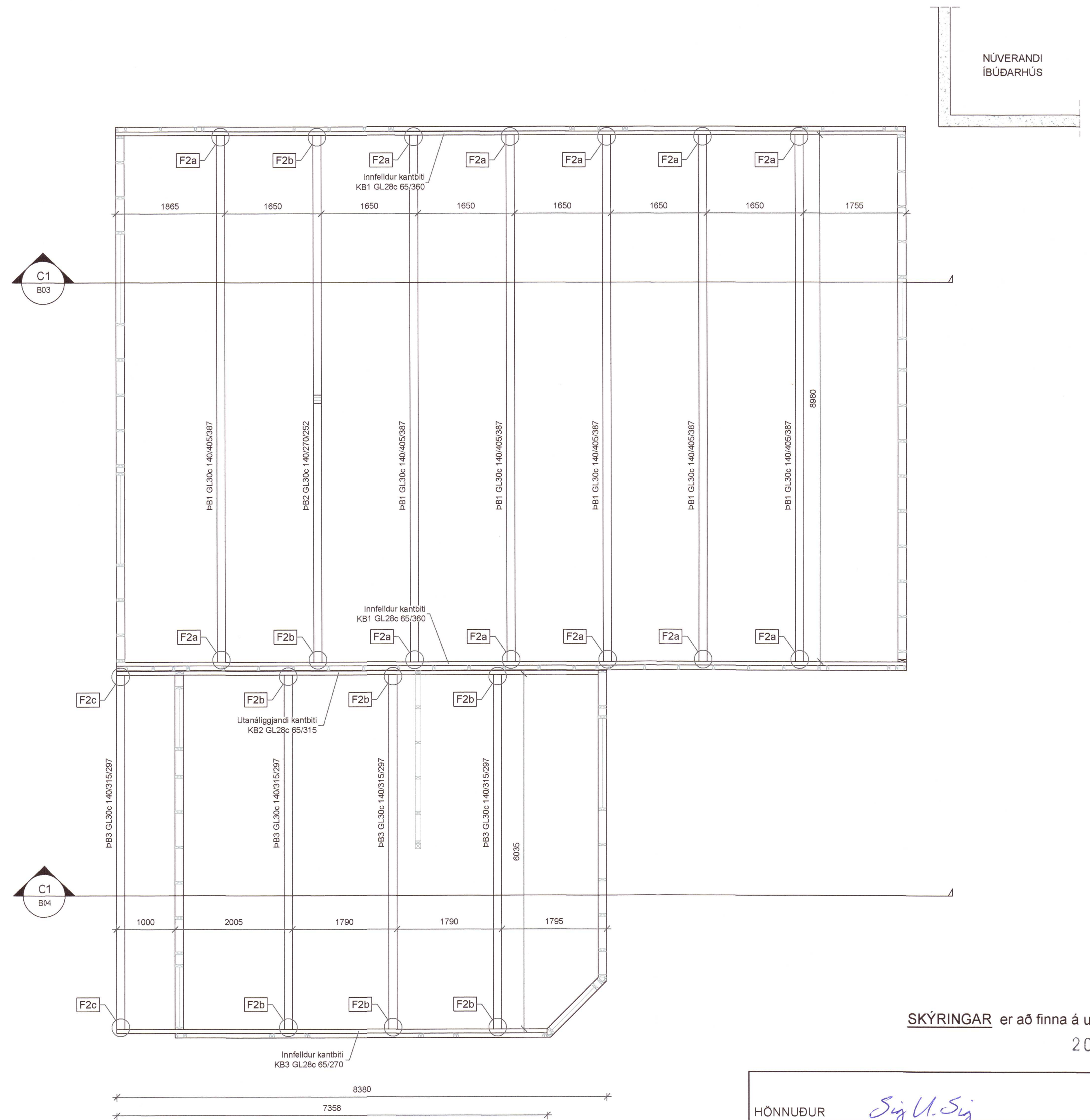
GRUNNMYND ÞAKVIRKI Mkv. 1:50
