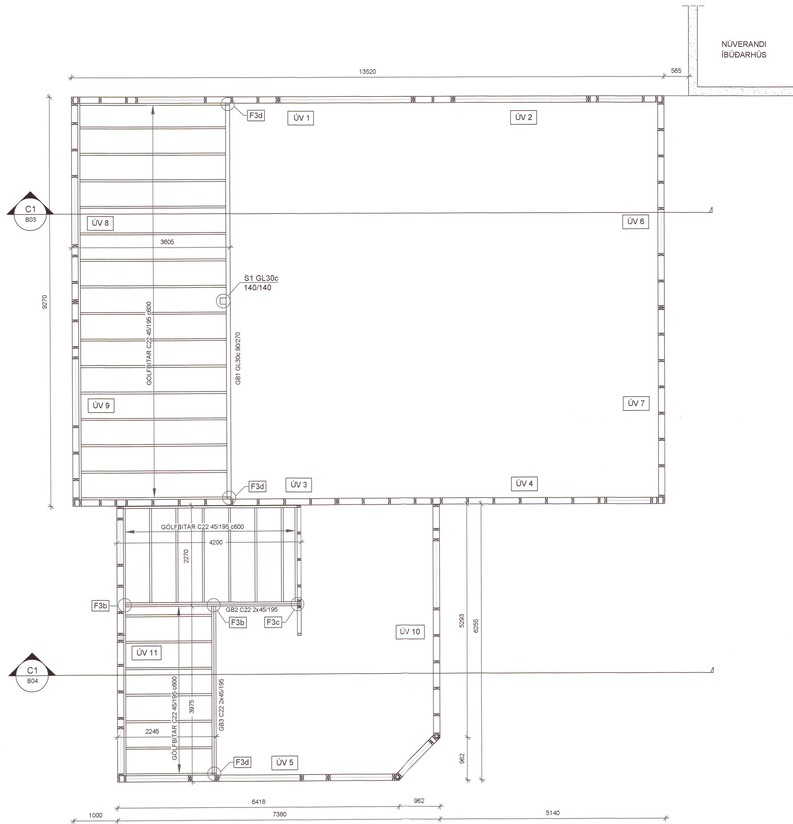
GRUNNMYND VEGGIR OG MILLILOFT Mkv. 1:50
