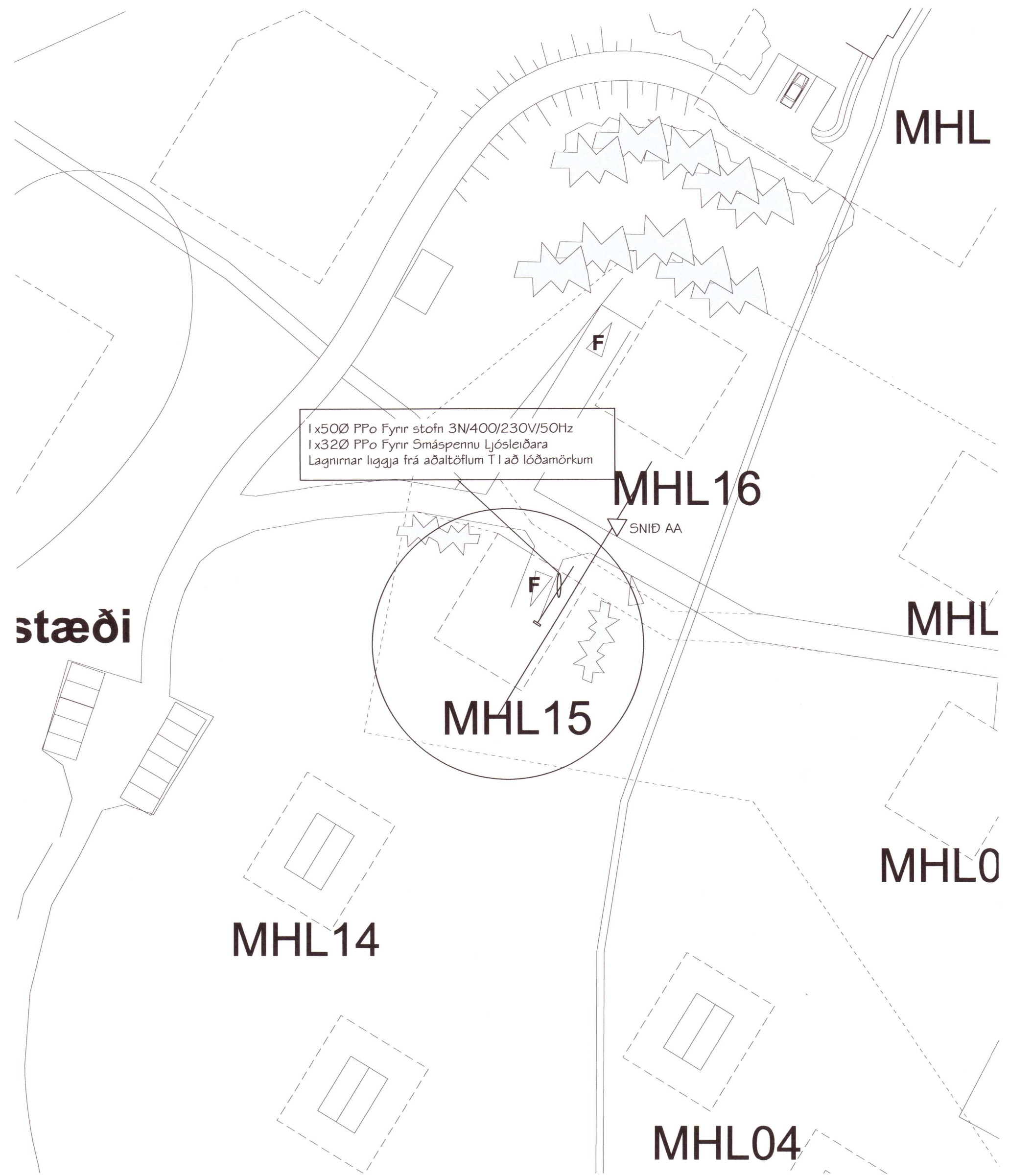
AFSTÖÐUMYND 1:500
