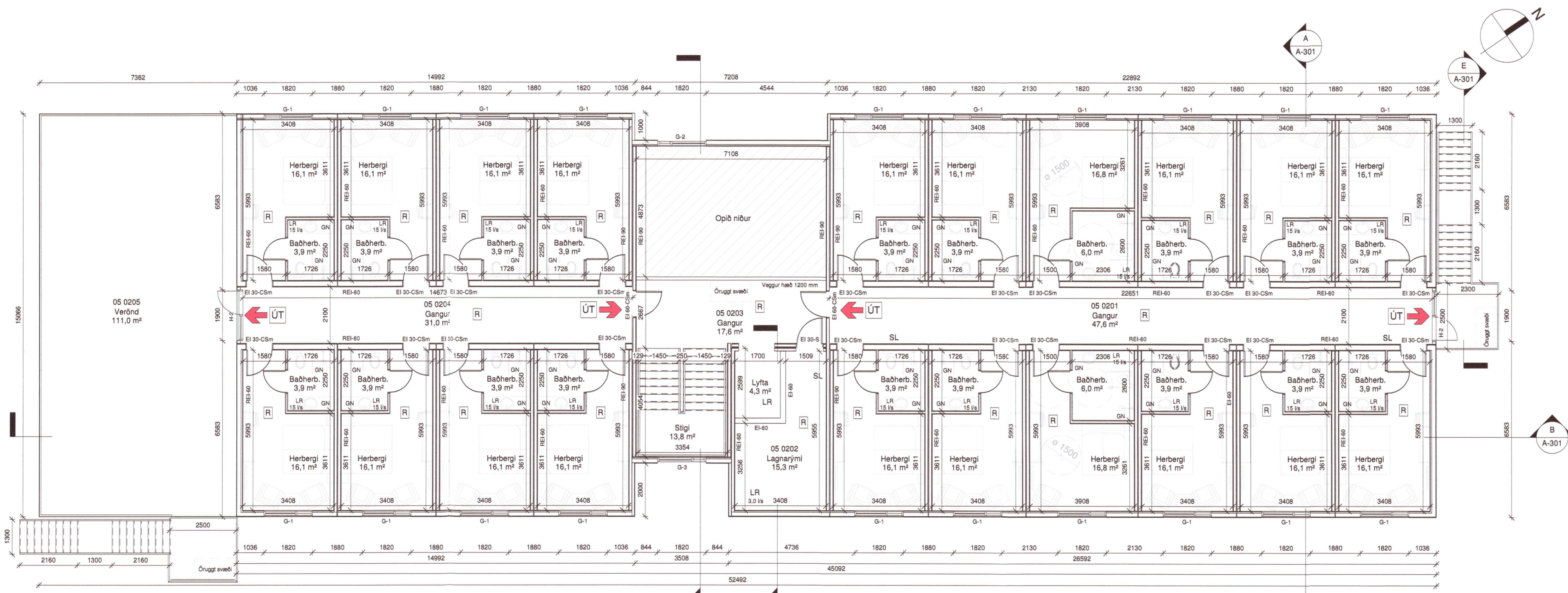
Grunnmynd 2. hæð 1 : 100
