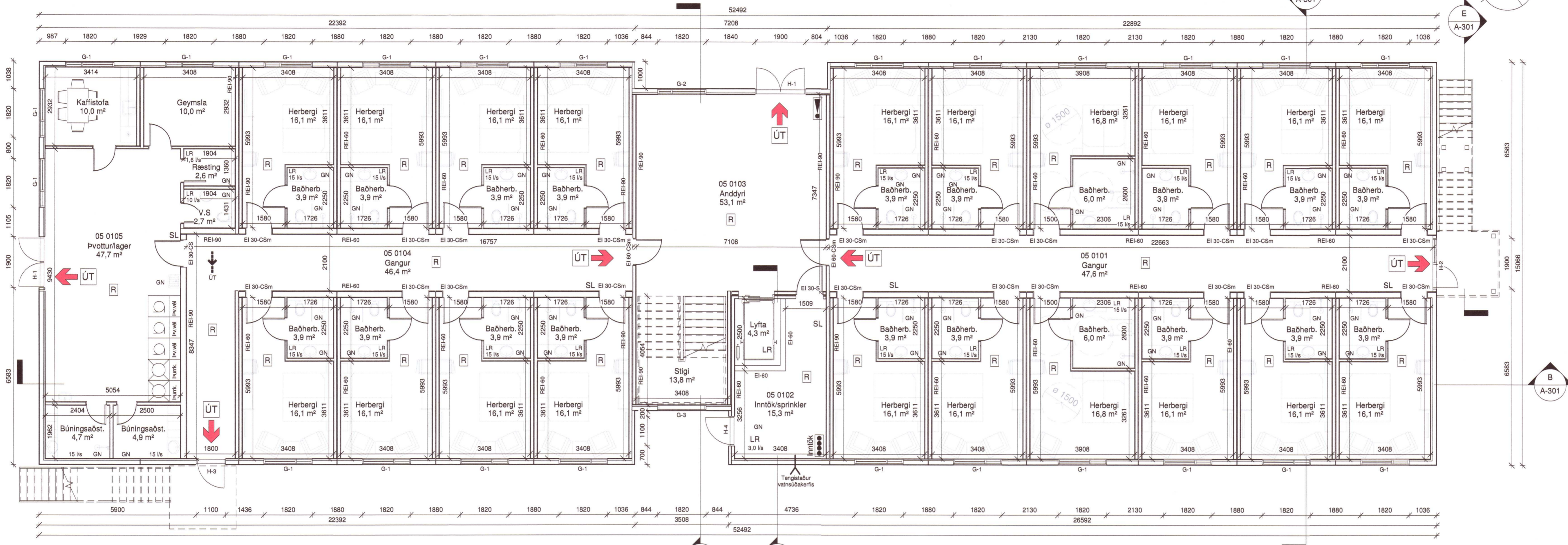
Grunnmynd 1. hæð 1 : 100
