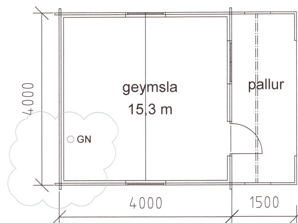
GRUNNMYND
