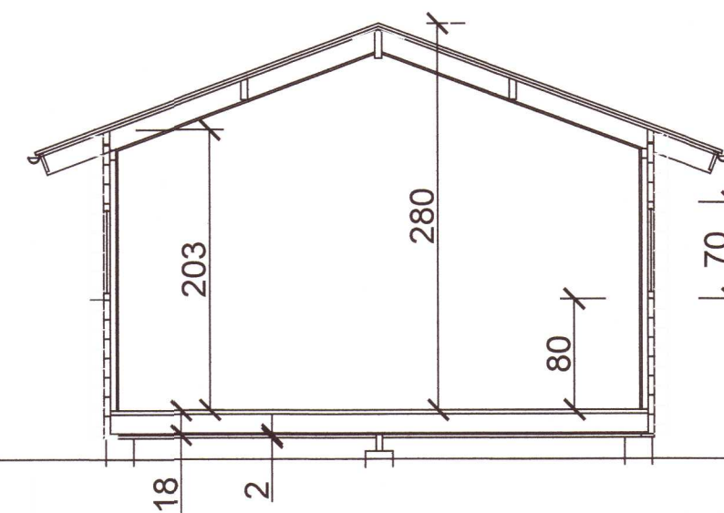
ÞVERSNIÐ
