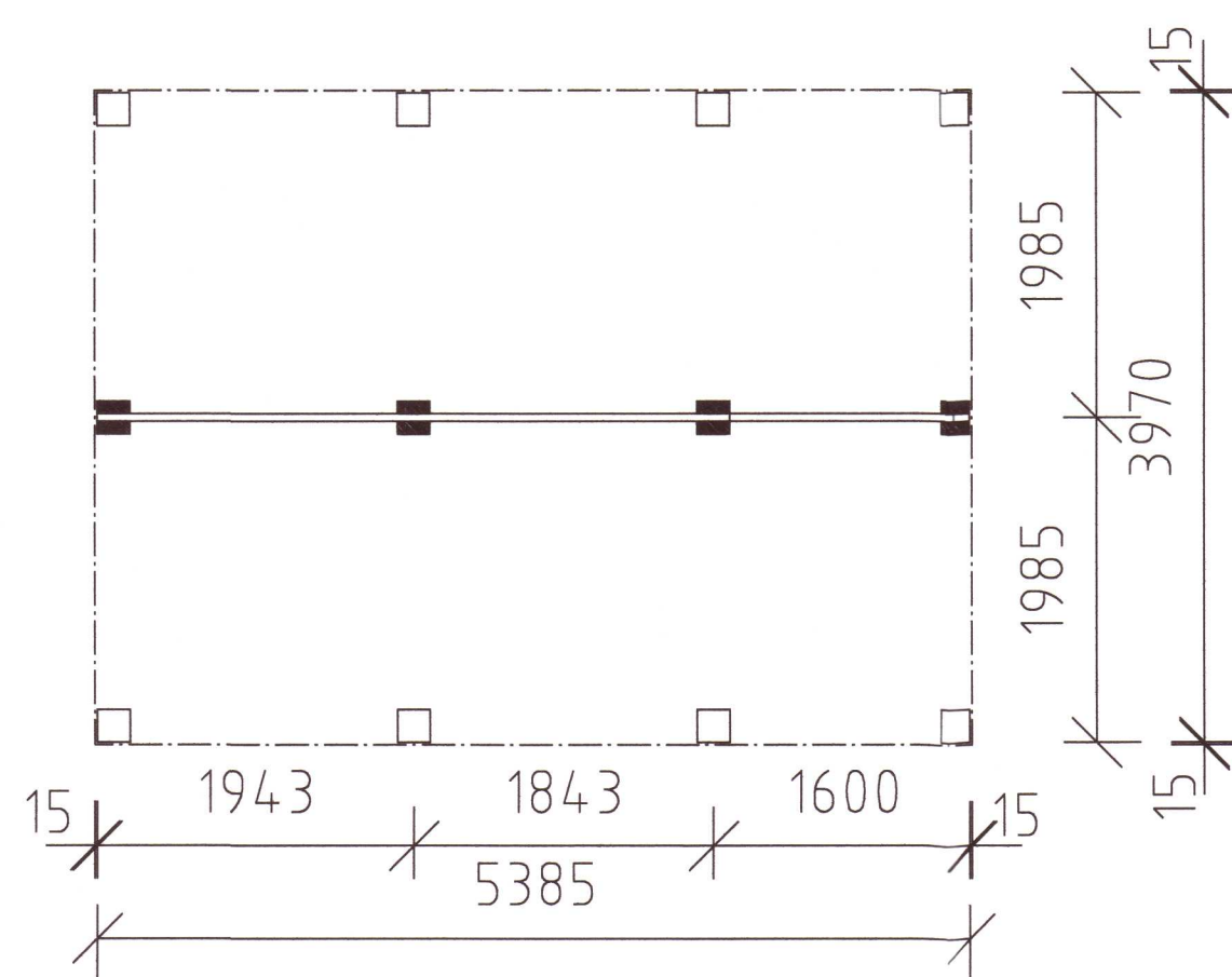
GRUNNMYND UNDIRSTÖÐUR
