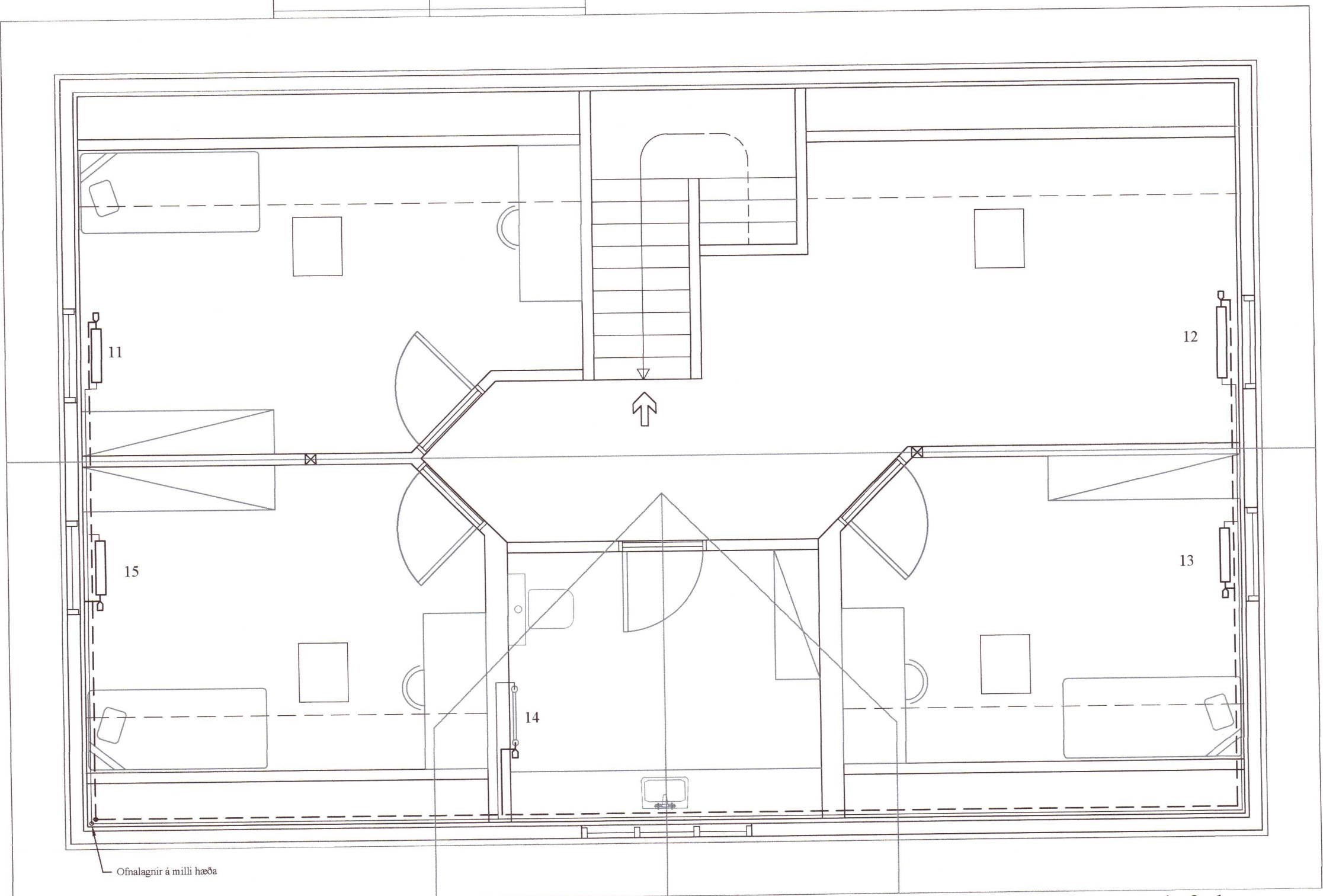
Grunnmynd ofnalagna MKV: 1:50
