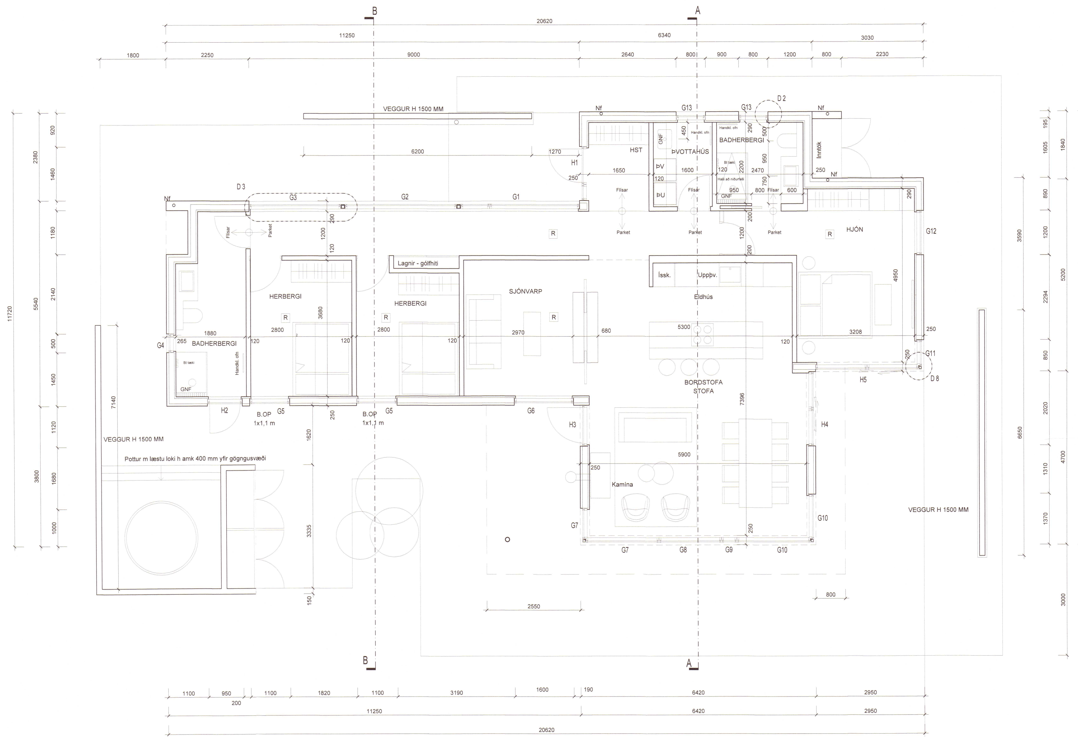
Grunnmynd 1:50
