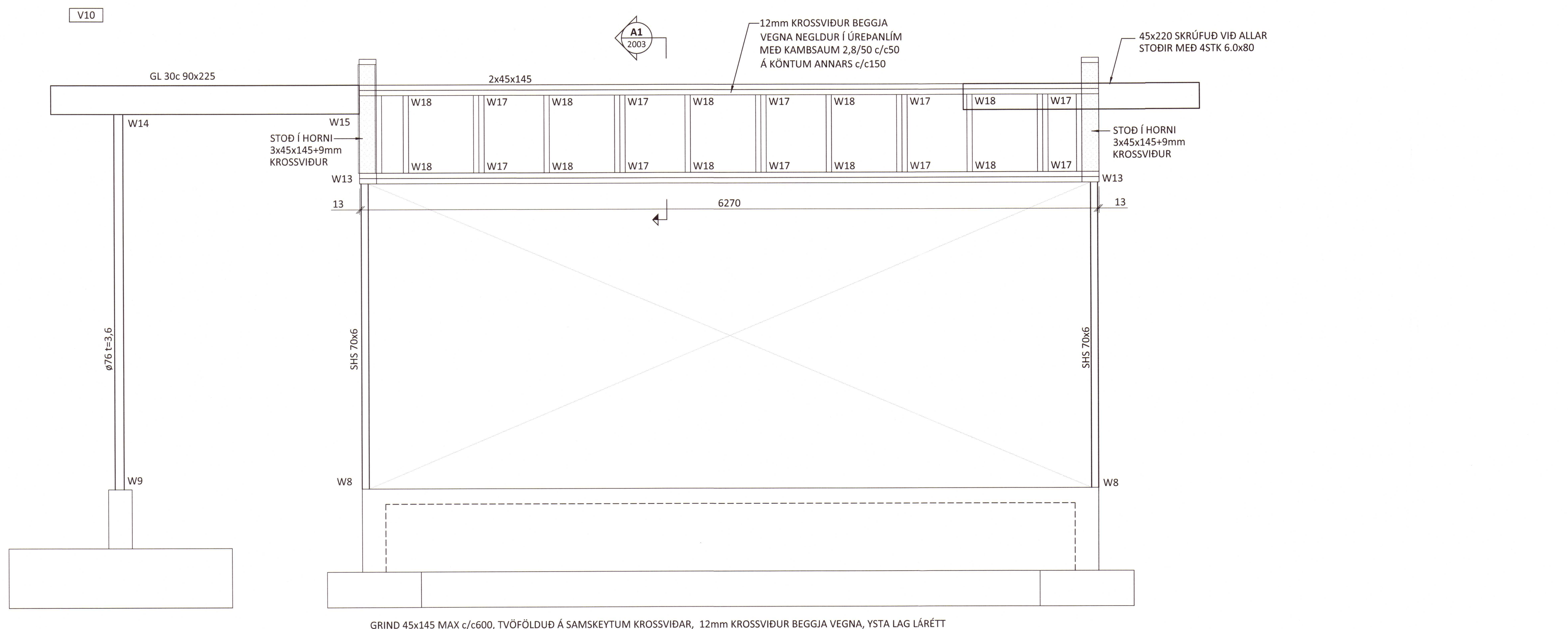
GRIND 45x145 MAX c/c600, TVÖFÖLDUÐ Á SAMSKYEYTUM KROSSVIÐAR, 12mm KROSSVIÐUR BEGGJA VEGNA, YSTA LAG LÁRÉTT
