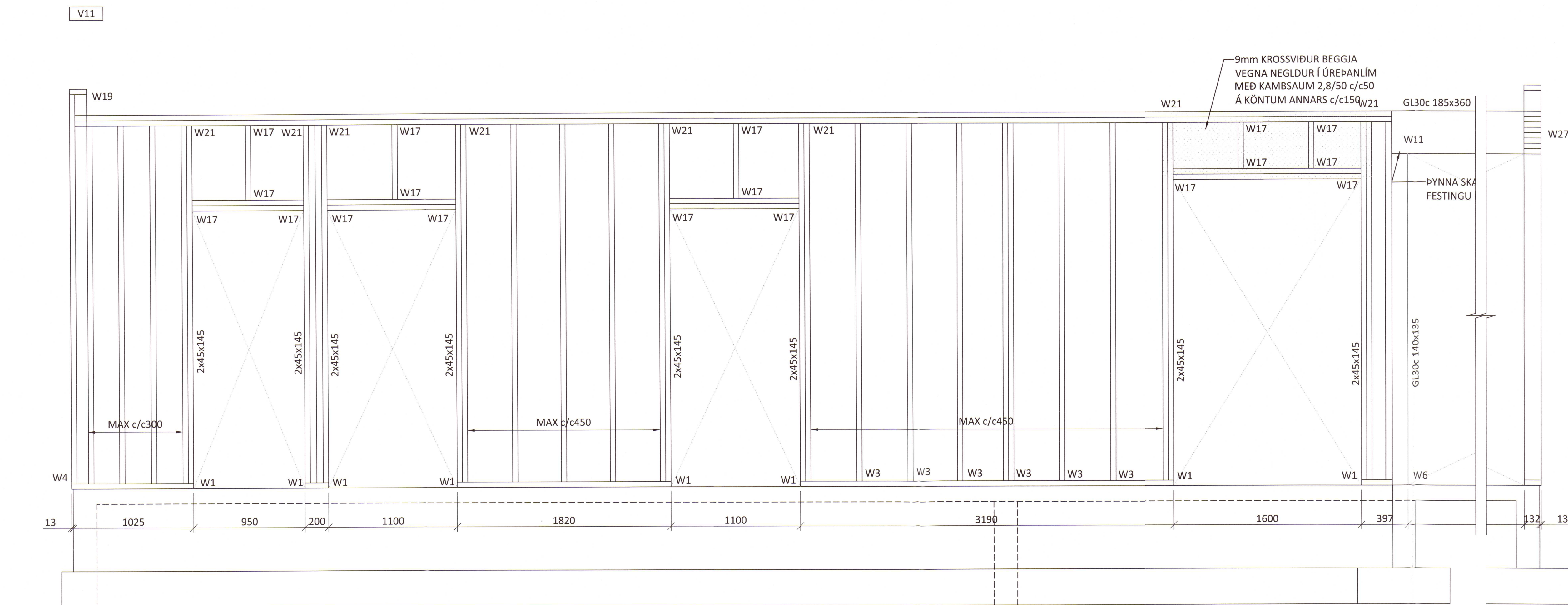
GRIND 45x145, 9mm KROSSVIÐUR AÐ UTAN NEMA Á BITA
