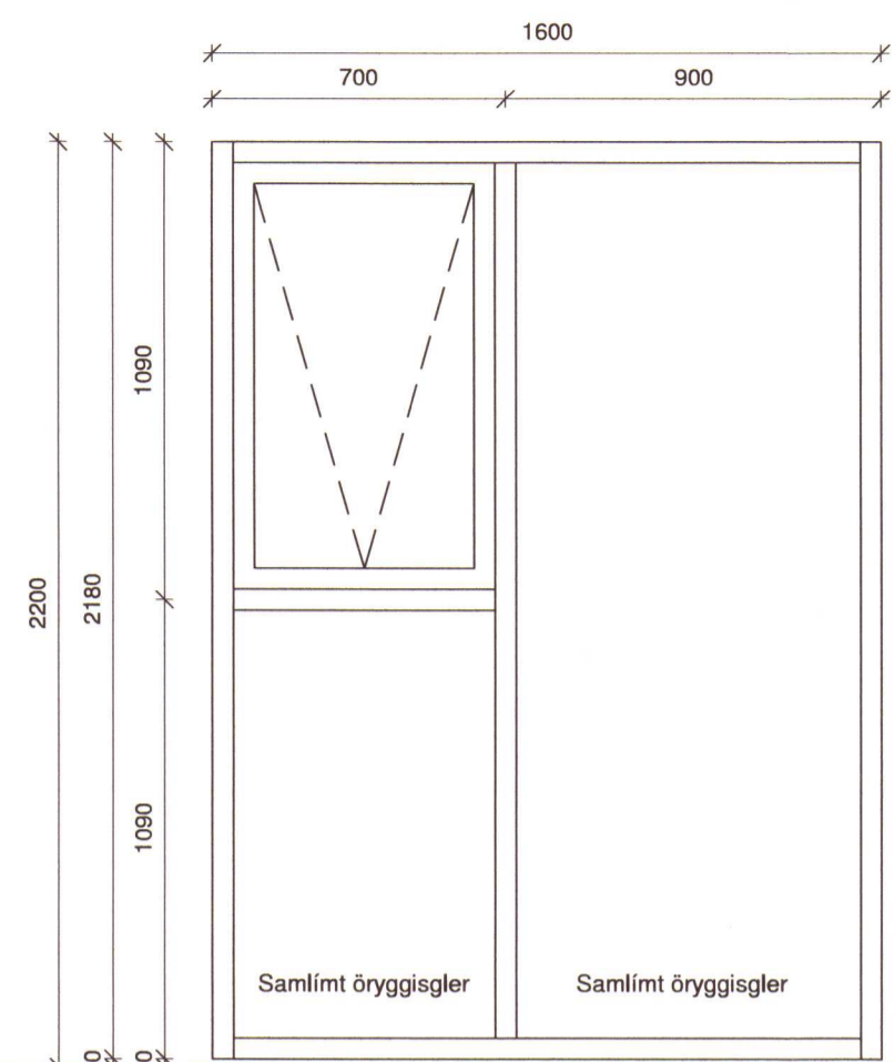
G-2 Hæð ofan á glugga frá botnplötu.....2200 mm Fjöldi.....1 stk
