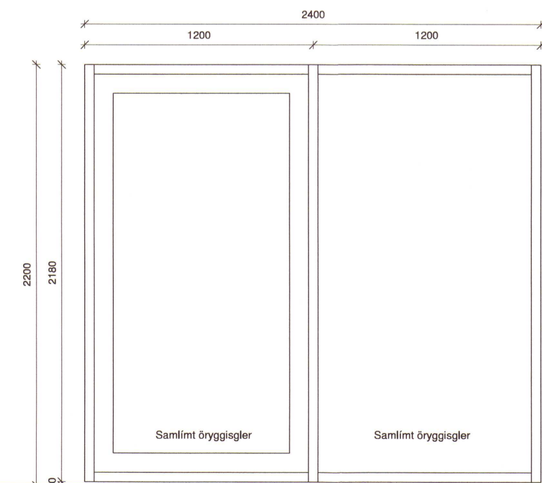
H-2 Hæð ofan á hurð frá botnplötu.....2200 mm Opnun.....Hægri hliðar Fjöldi.....1 stk
