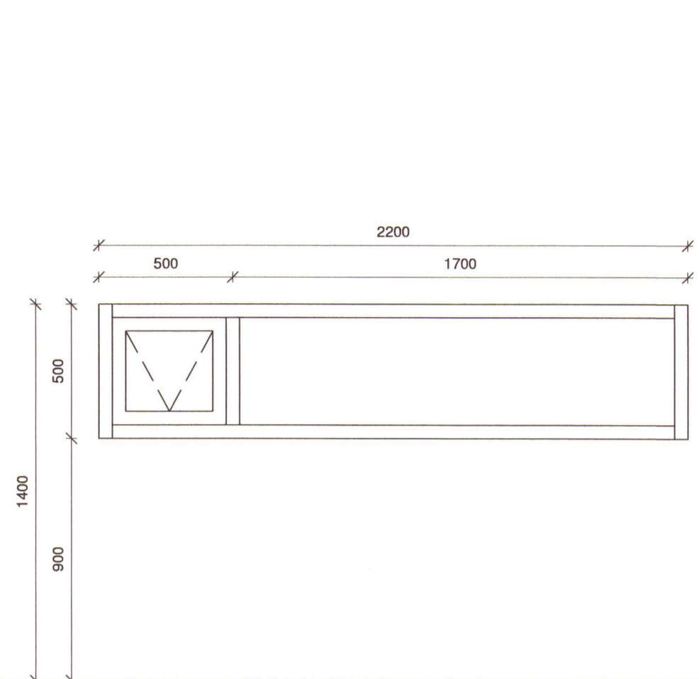
G-1 Hæð ofan á glugga frá botnplötu.....2200 mm Opnun.....Toppengt Fjöldi.....1 stk
