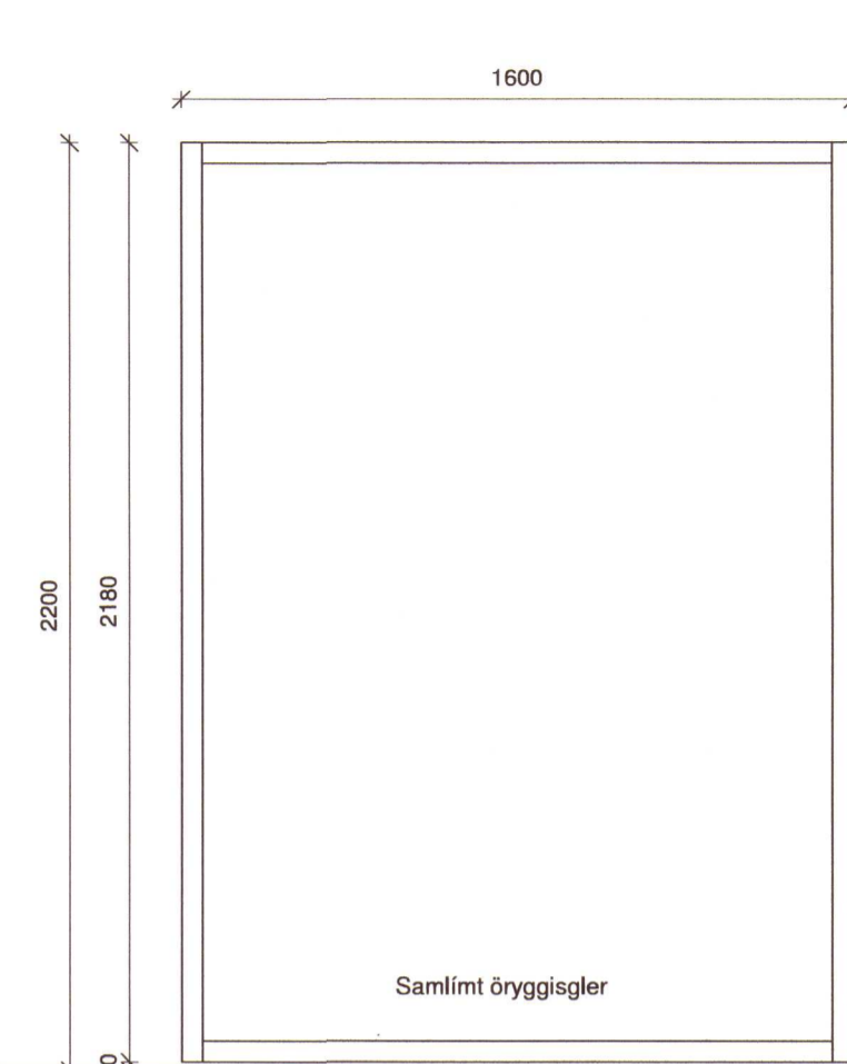
G-3 Hæð ofan á glugga frá botnplötu.....2200 mm Fjöldi.....1 stk
