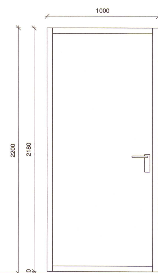
H-1 Hæð ofan á hurð frá botnplötu.....2200 mm Opnun.....Hægri inn Fjöldi.....1 stk
