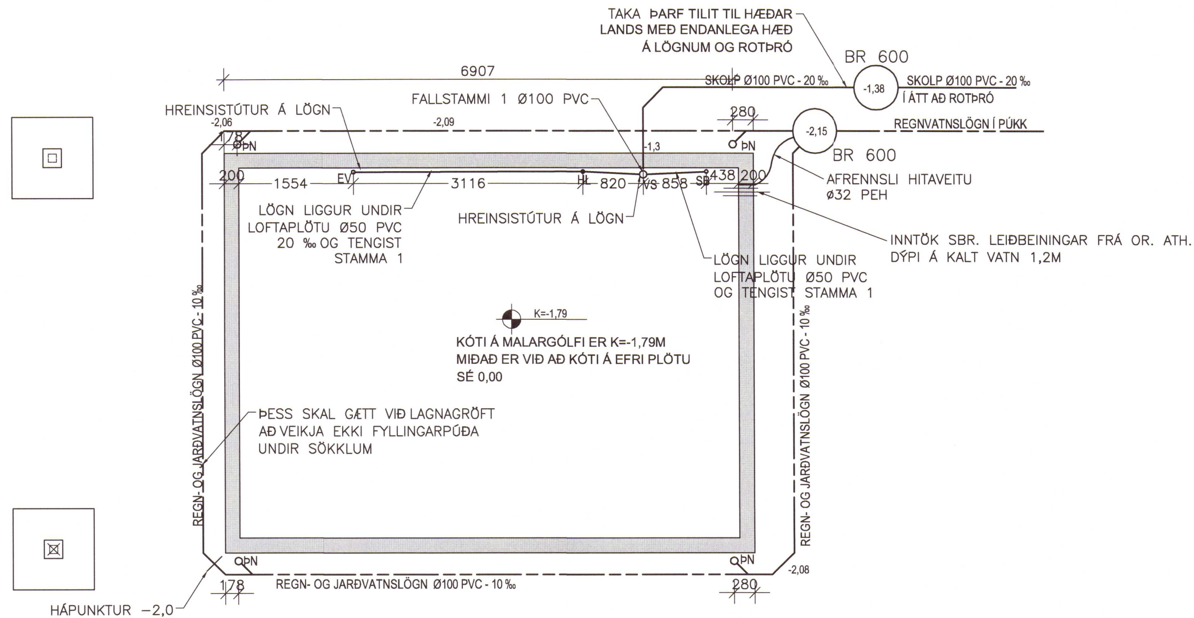
GRUNNMYND KJALLARA GRUNNLAGNIR 1:50
