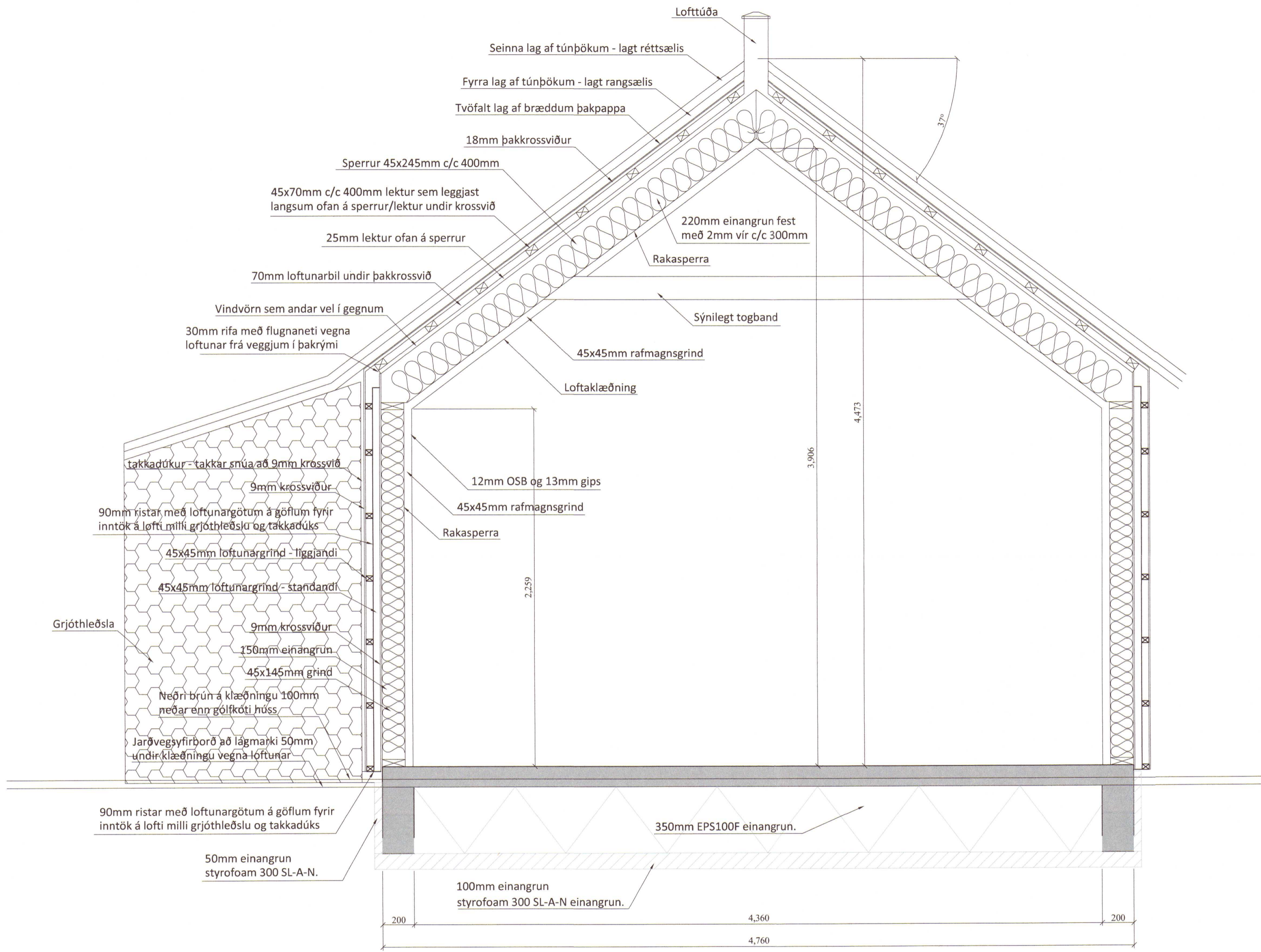
Snið mkv. 1:20
