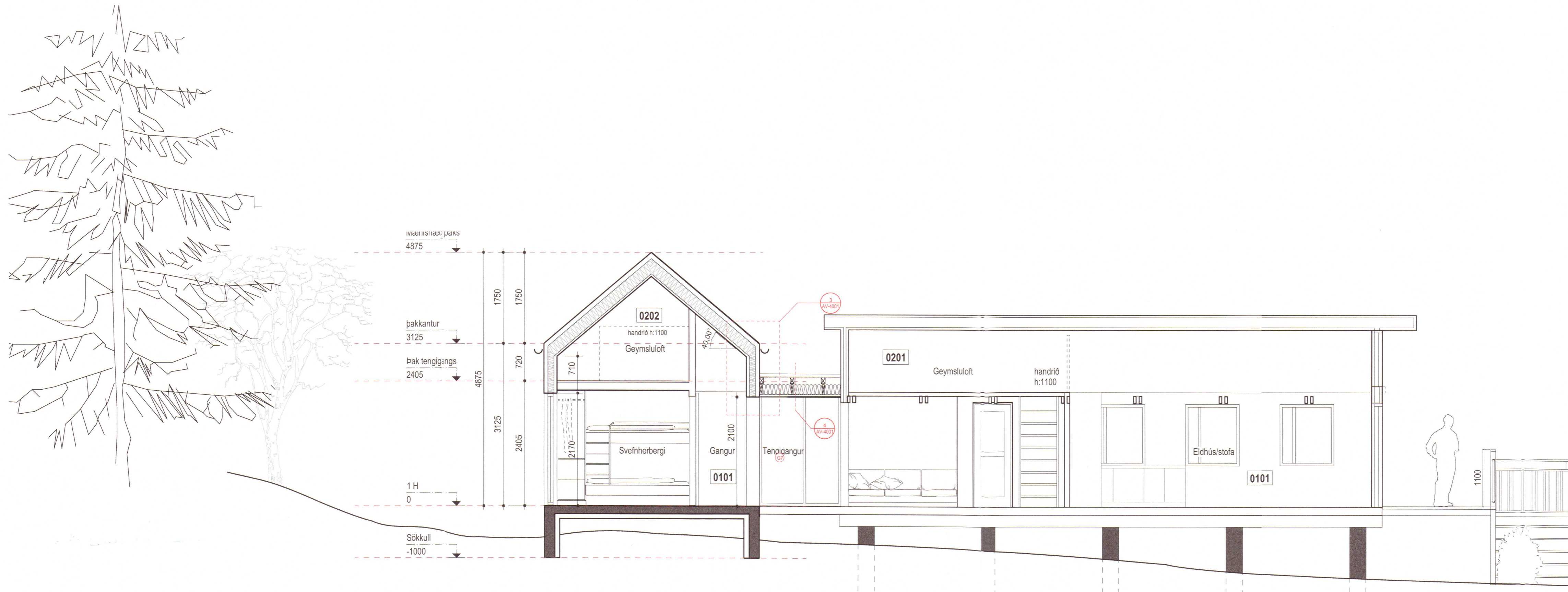
2 Austurhlíð - Sneiðing B 1:50
