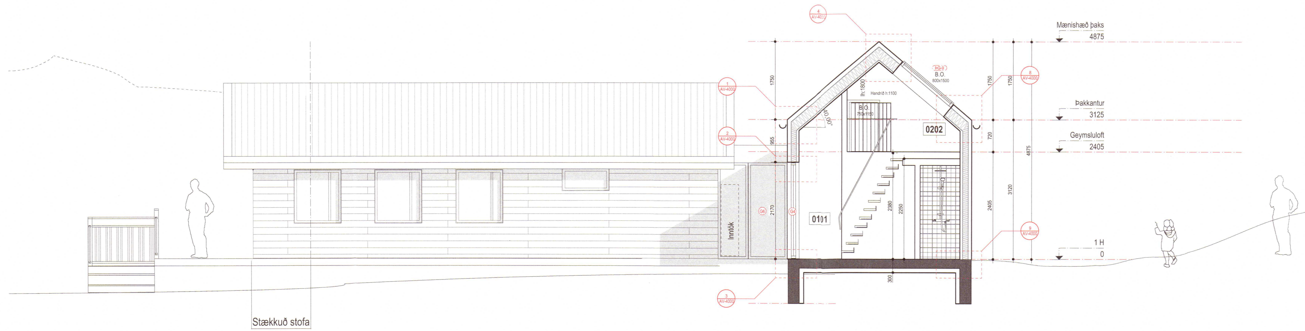
3 Suðurhlíð - Sneiðing A 1:50
