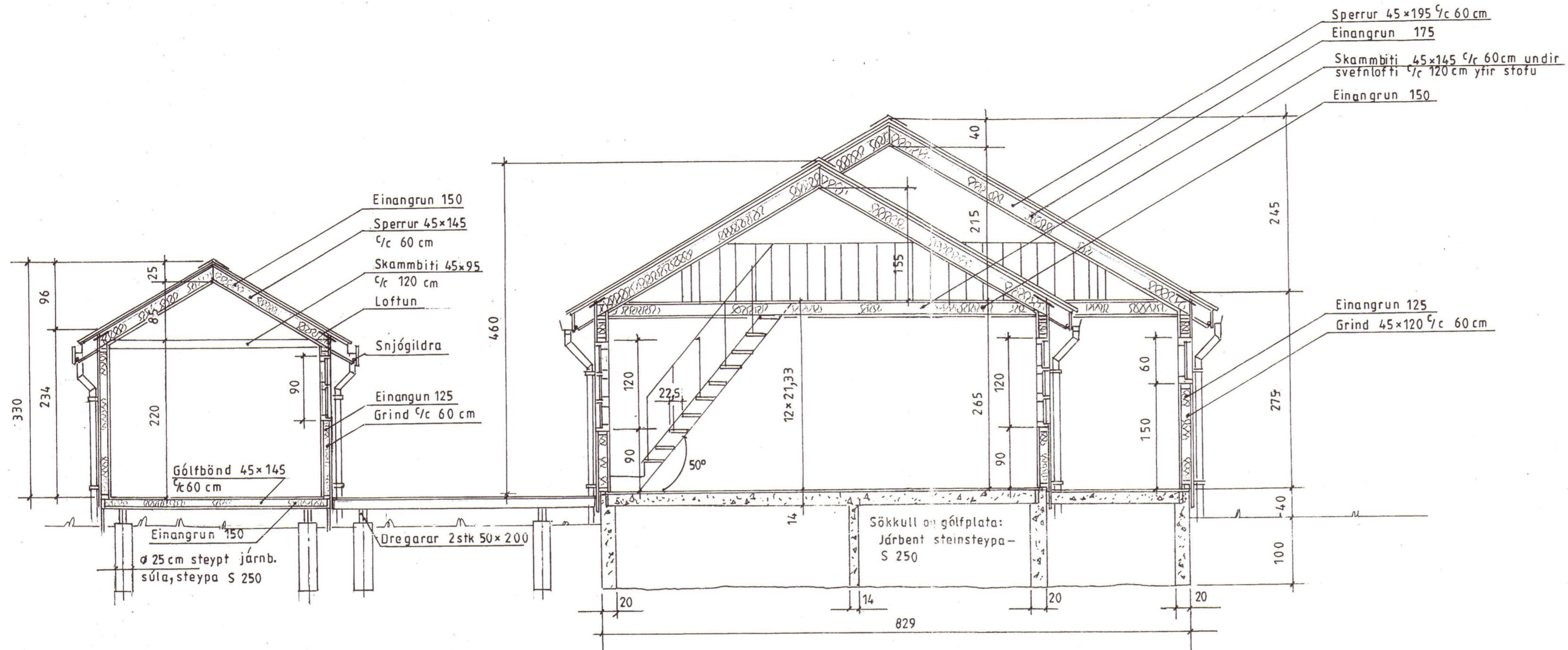
Sníð A-A
