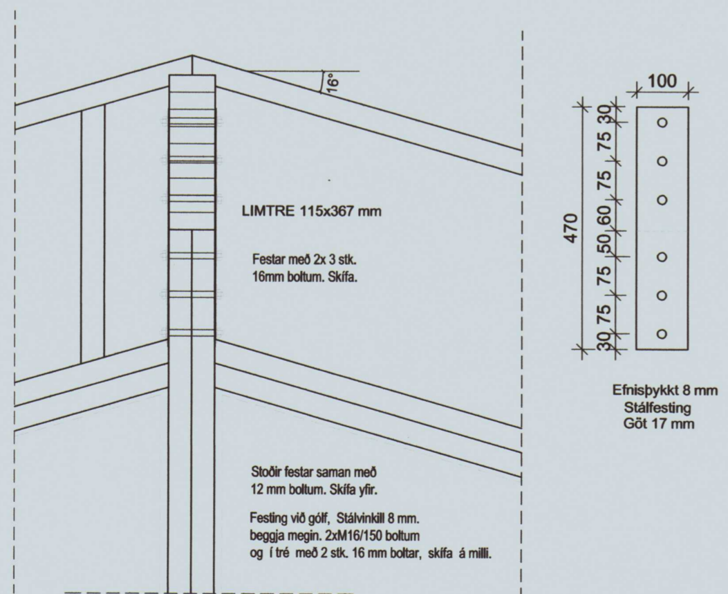
F Festing límtré Mkv. 1:10
