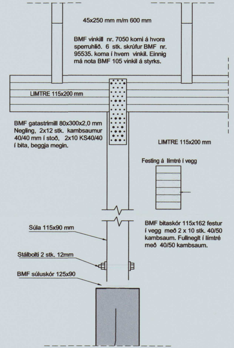
G Súla undir þakskyggni 1:10
