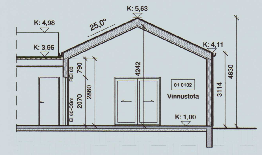
Snið D-D 1 : 100
