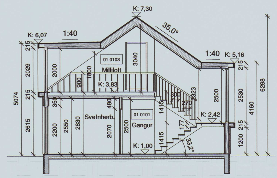
Snið A-A 1 : 100
