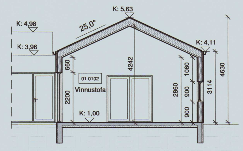
Snið C-C 1 : 100
