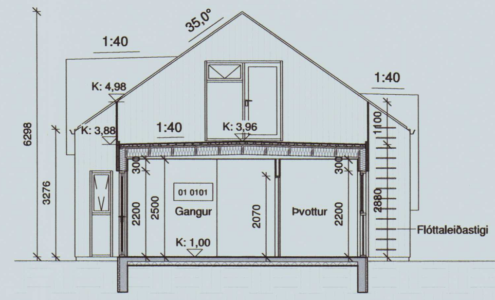
Snið B-B 1 : 100
