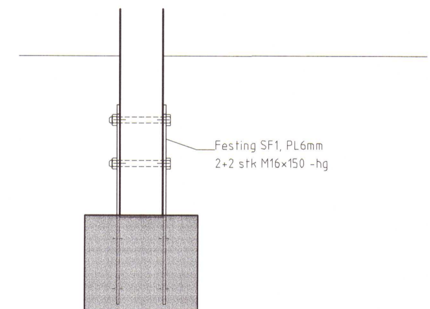
Sérmynd S6 1:10
