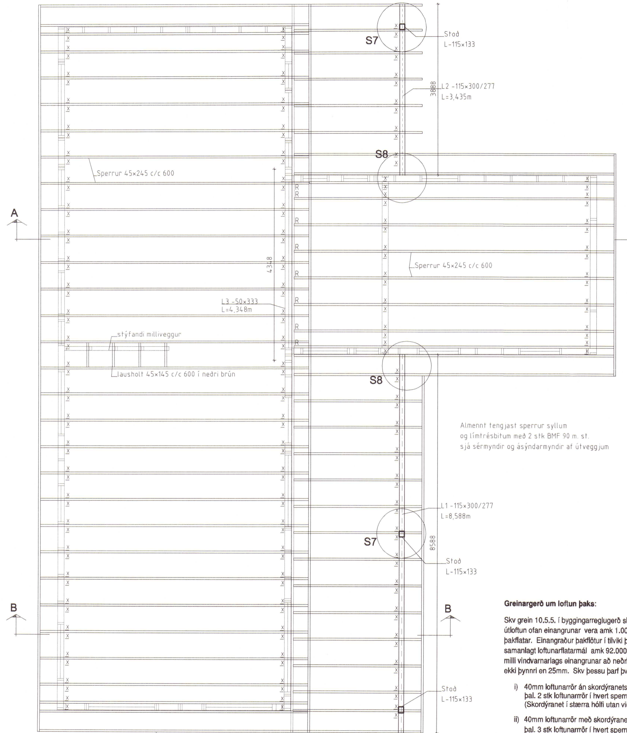
Þakmynd 1:50
