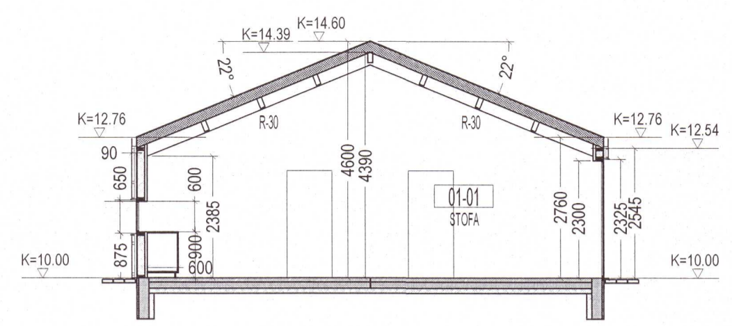
SNEIÐMYND A, MKV. 1:100
