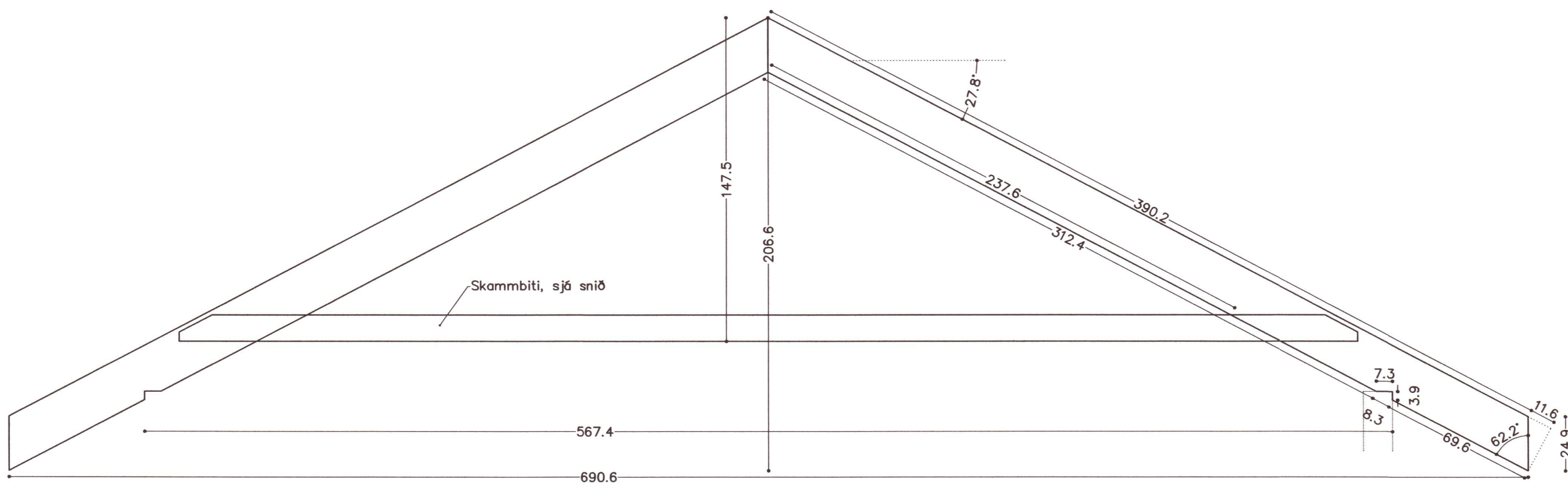
Þaksperrur 1:20
