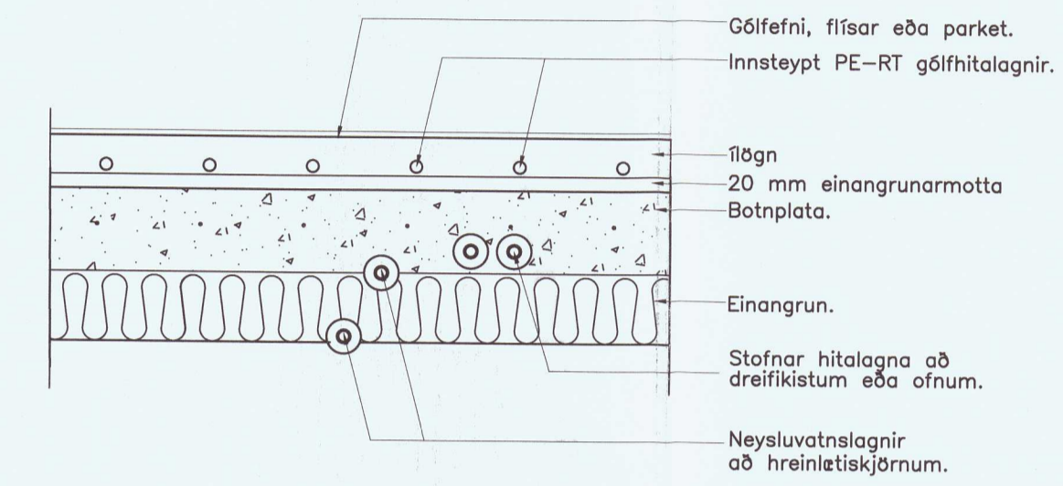
Snið í gólf íbúðahúss. 1:10.
