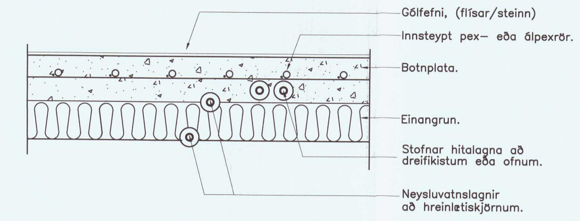
Snið í gólf bílskúrs. 1:10.
