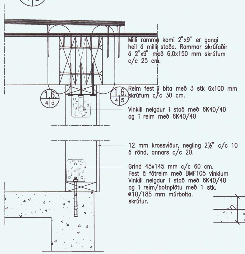
1.3 Sérmynd 1.3. 1:10.
