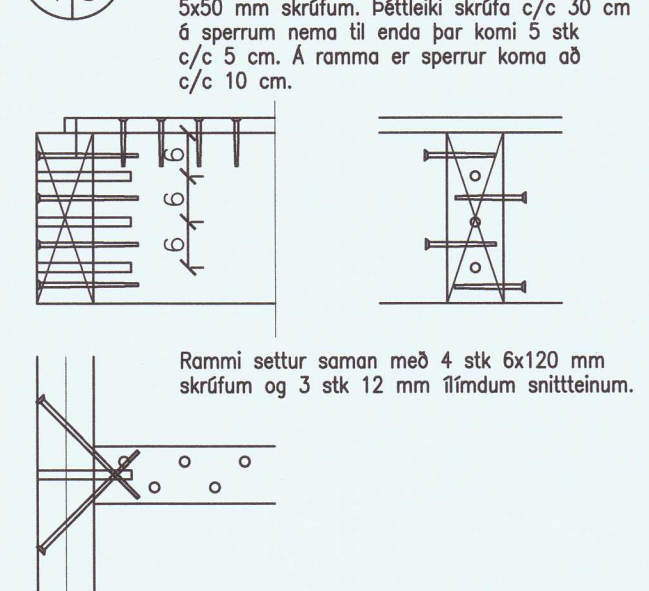
1.6 Sérmynd 1.6. 1:10.
