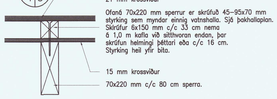
1.5 Sérmynd 1.5. 1:10.
