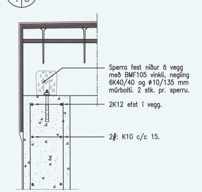
1.1 Sérmynd 1.1. 1:10.
