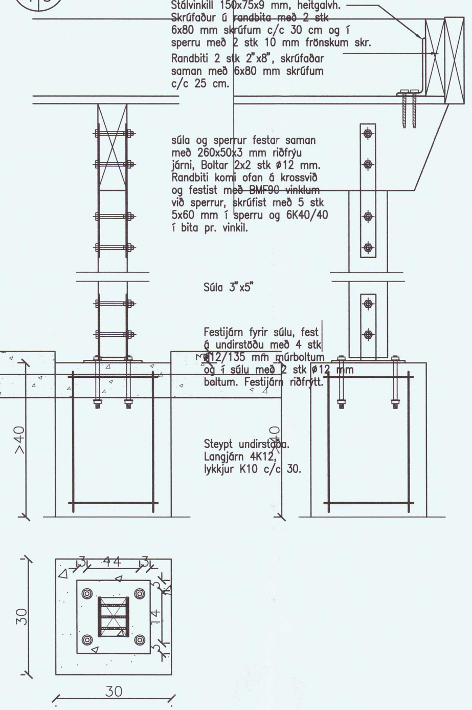
1.4 Sérmynd 1.4. 1:10.
