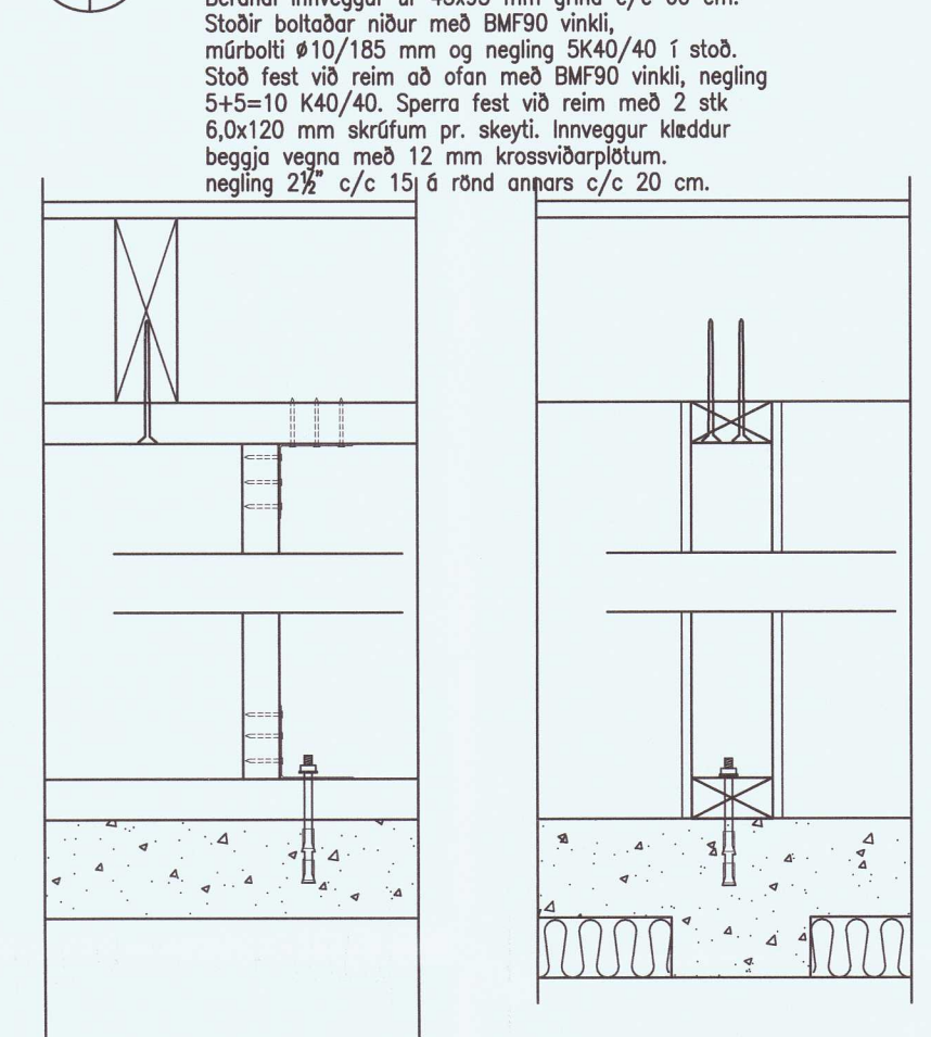
1.7 Sérmynd 1.7. 1:10.
