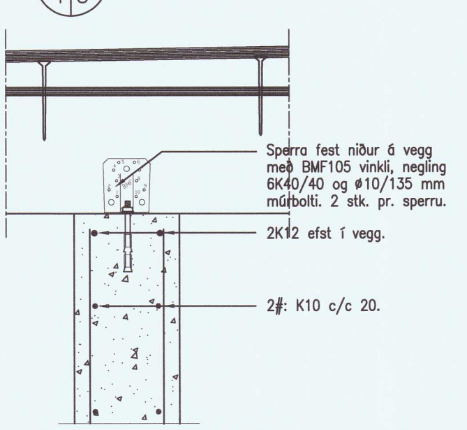
1.2 Sérmynd 1.2. 1:10.
