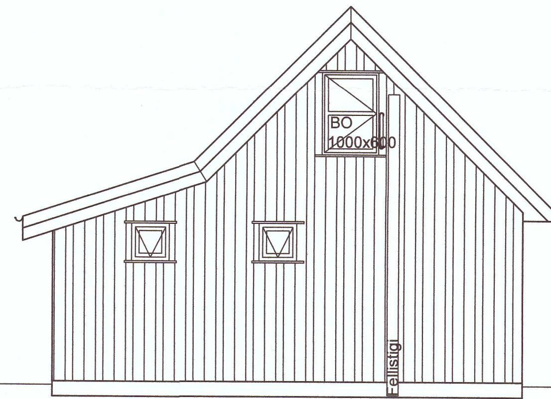
Norður 1:50
