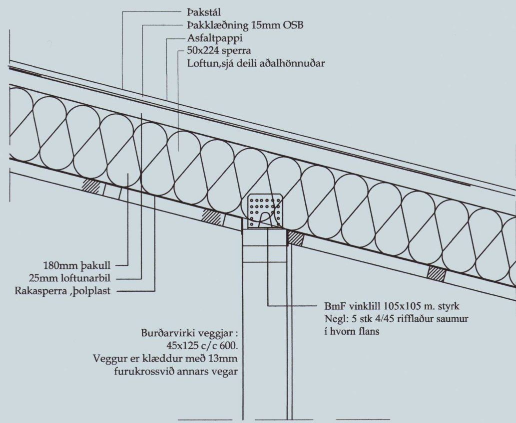
Snið C mk. 1:10
