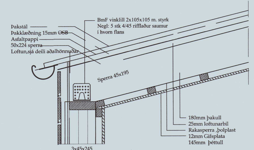
Snið E mk. 1:10
