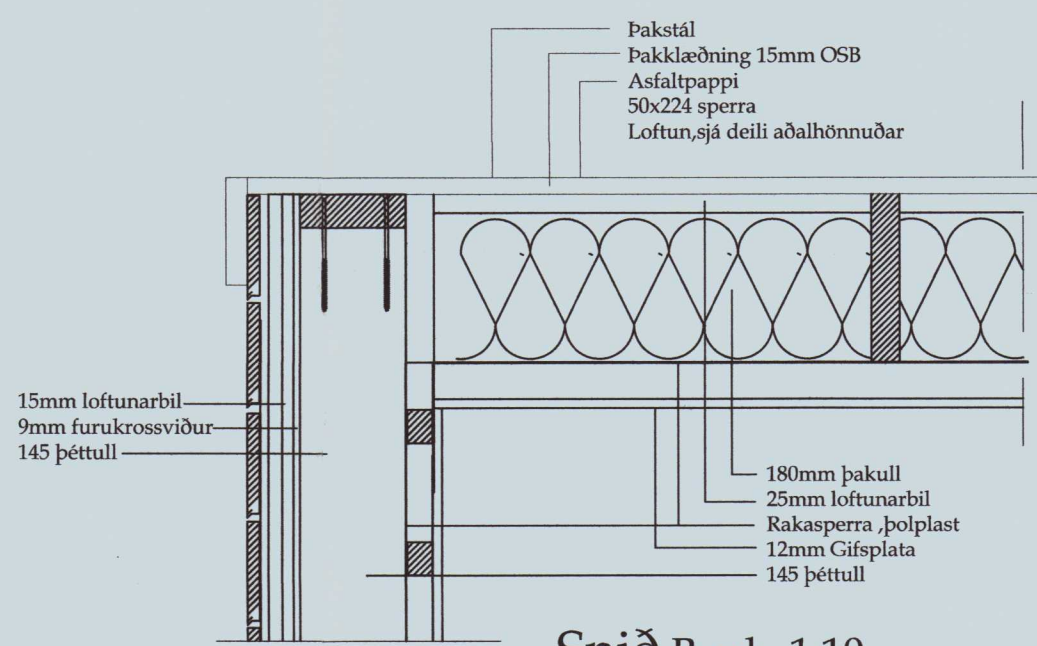
Snið B mk. 1:10
