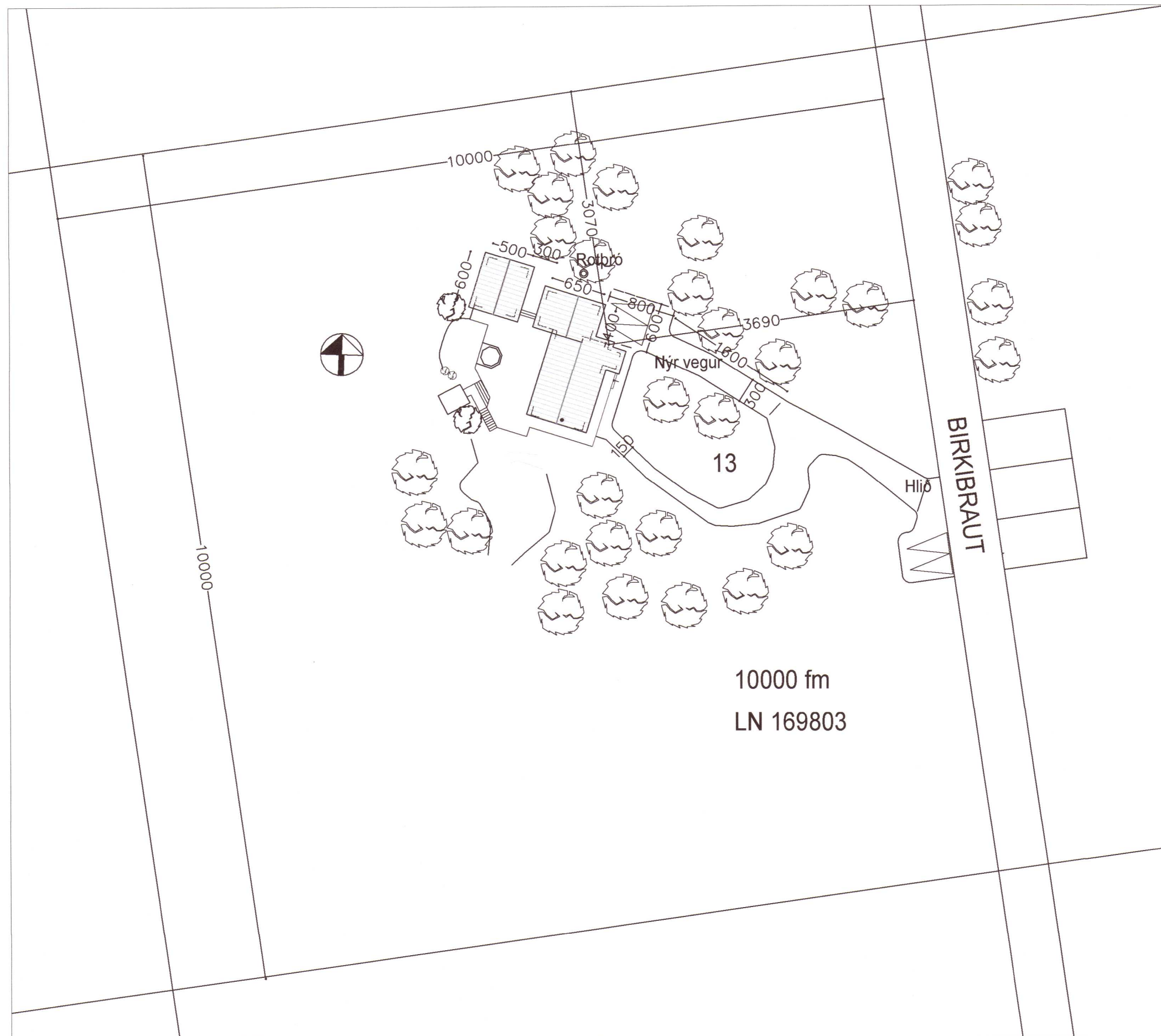
AFSTÖÐUMYND 1:500
